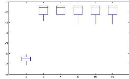
Maximin LHS
