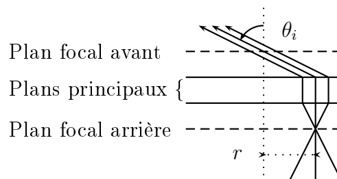
FIG. A.2 – Schéma de l'objectif
