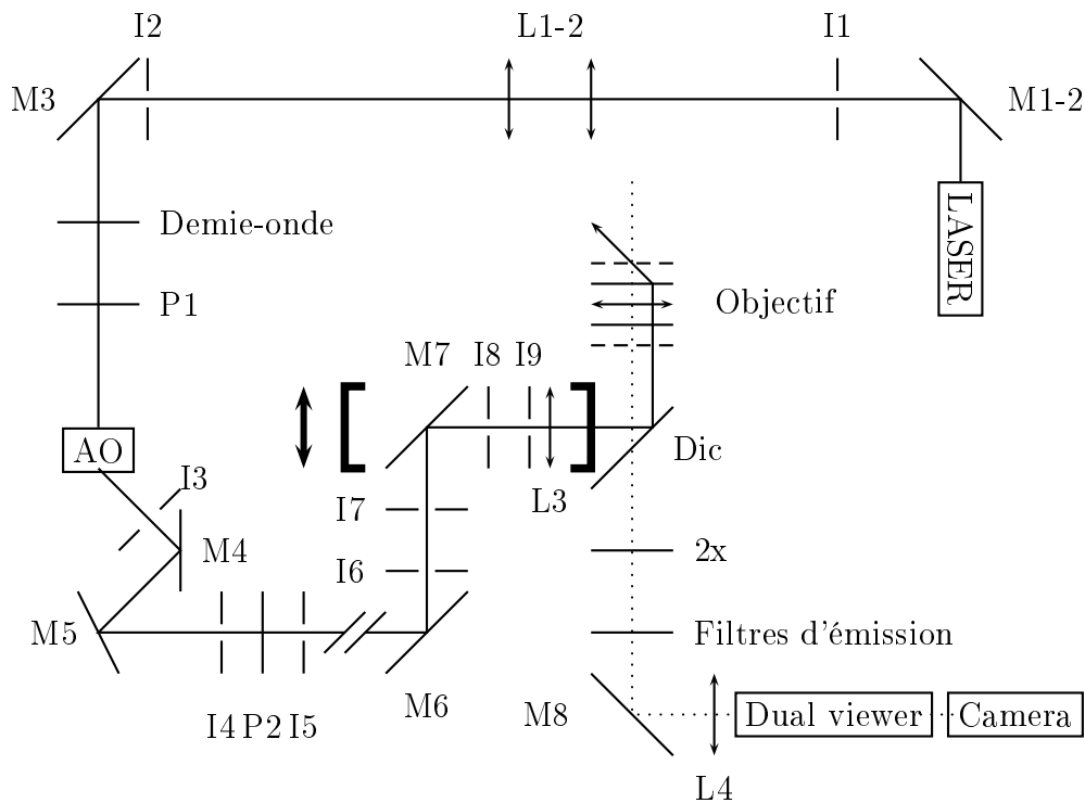
FIG. A.1 – Schéma du microscope
