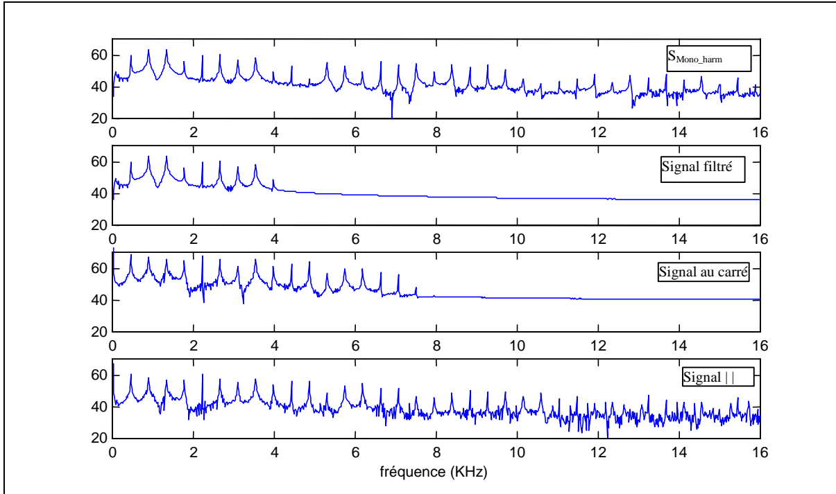
Figure 4.19 : Effets des non-linéarités sur un peigne de sinus
