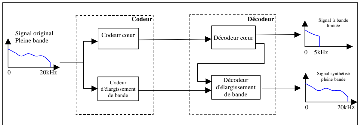
Figure 1.2 : Système d'enrichissement de spectre
