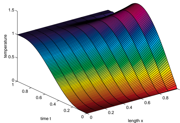
FIG. 10. Planification de trajectoire à partir d'une fonction Gevrey d'ordre 2.5.
