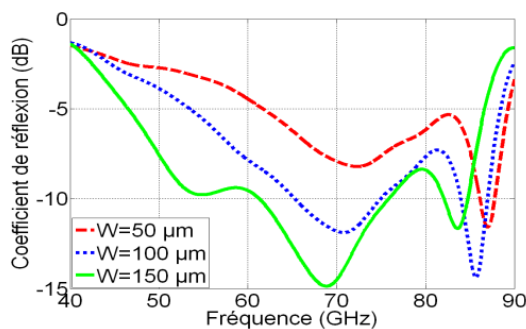
Figure 2 : Effet de Changement de largeur de brins sur S11
