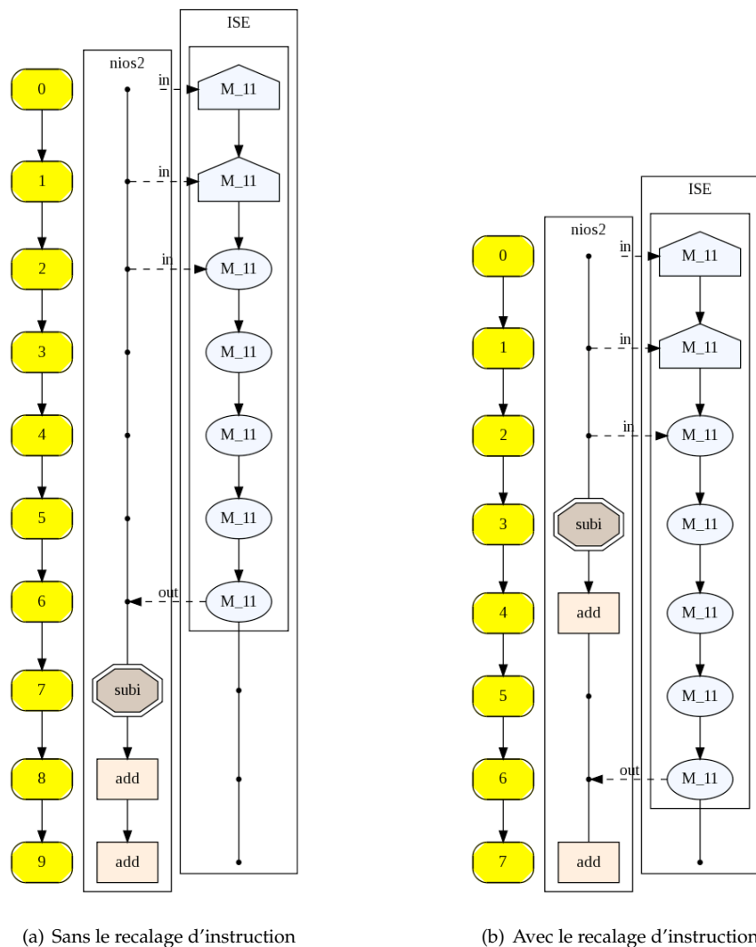
FIG. 9 – Exemple d'ordonnement du graphe de la figure 7(c) et de placement sur le modèle d'architecture B
