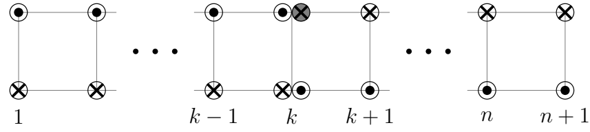
Modèle 2 de schéma de piquage
