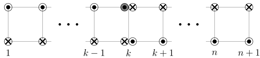
Modèle 3 de schéma de piquage
