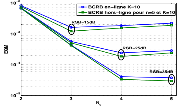
FIG. 2 – BCRB en fonction de N_c pour f_dT = 0.5 et RSB = 15dB , 25dB et 35dB
