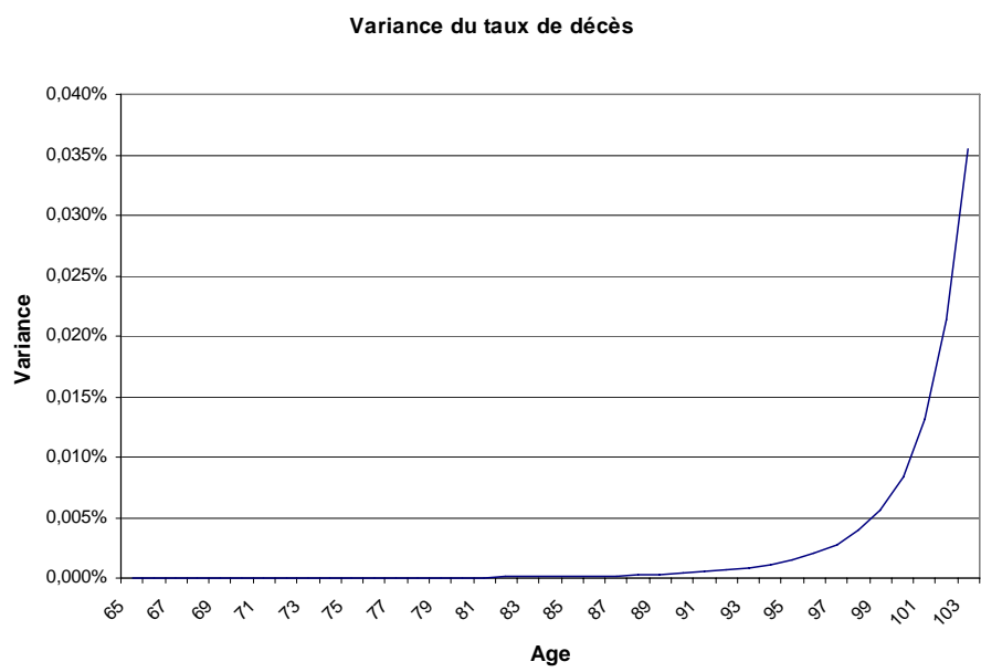
Fig. 3 : Variance du taux de décès avec l'âge
