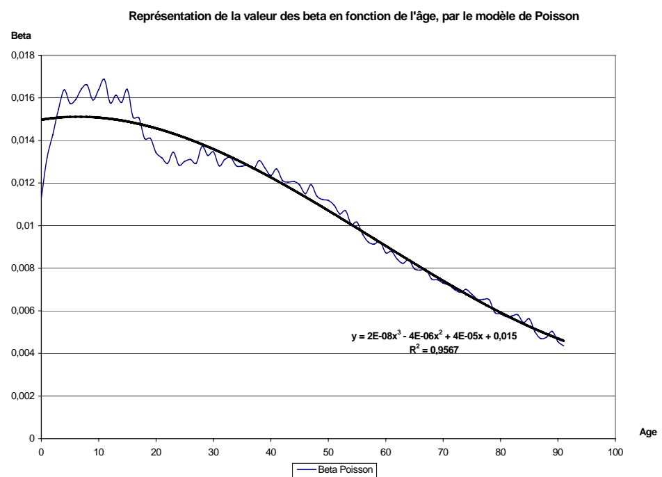
Fig. 7 : Approximation polynomiale des paramètres bêta obtenus par les modèles log-poisson.
