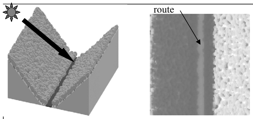
Figure 6 : a) Maquette de vallée. b) Simulation DART d'image de télédétection. Simulation réalisée dans le cadre de la préparation du système Pléiades du CNES.
