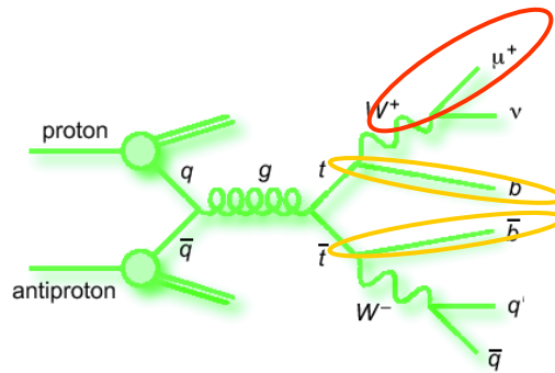
Fig. 5 : Schéma de théorique (Feynman) de la collision proton-antiproton produisant des quarks top.
