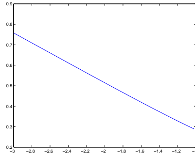
Fig. 16. \frac{1}{\|u^\varepsilon\|_{H^1(O_\varepsilon)}^2} = f(\log_{10} \varepsilon)
