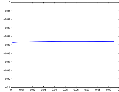
Fig. 18. \|u^\varepsilon\|_{L^2(O_\varepsilon)} = f(\varepsilon)
