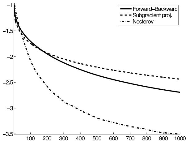
FIG. 2 – Décroissance avec k de l'erreur \log_{10}(\|f^{(k)} - f^*\|/\|f^*\|) pour l'algorithme dual avec itération explicite-implicite (trait plein), avec itérations de Nesterov (trait plein-pointillés) et par projection de sous-gradient [4] (trait en pointillés), avec \tau = \|f_0\|_{TV}/4 .
