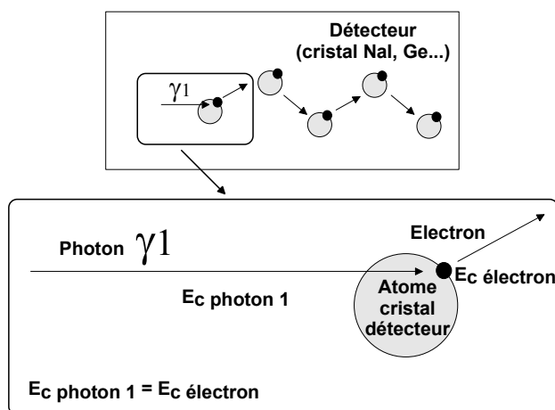
Figure 2.17 : Effet photoélectrique.
