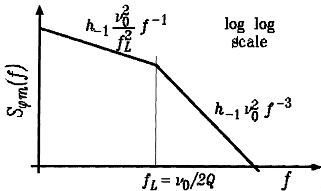
Fig. 4: Allure de la pente de la densité spectrale de bruit de phase mesurée sur une paire de résonateurs
