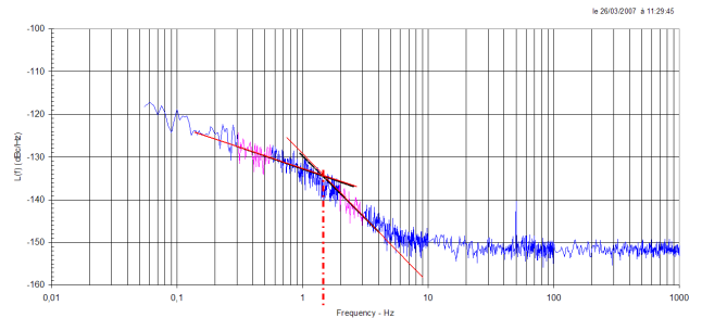
Fig. 5: Courbe de mesure du bruit de phase obtenue sur la paire de résonateurs (31,28)
