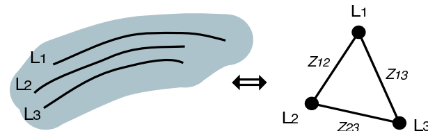
FIG. 8 – L’ensemble de lignes initial est représenté par un graphe où les lignes sont les noeuds et les zones de recouvrement sont les arêtes. La partition est obtenue en utilisant un algorithme de contraction d’arêtes jusqu’à ce qu’il n’y ait plus aucune arête dans le graphe.
