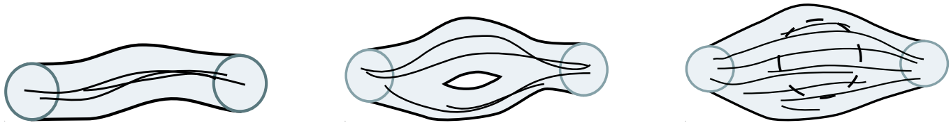
FIG. 4 – L'exemple de gauche possède une structure de ligne à \epsilon près : deux extrémités et un chemin unique à \epsilon près. Les deux autres exemples ne respectent pas ces contraintes : au milieu , la présence d'un trou implique l'existence de plusieurs chemins possibles ; à droite , la dilatation des lignes initiales par \epsilon est trop épaisse, aucun chemin à \epsilon près n'est donc présent.
