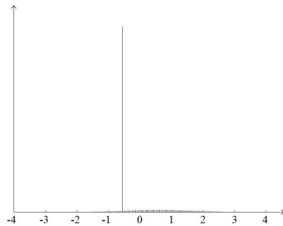
(F.a) \Delta(0, 1, \frac{2}{\sqrt{3}}, \frac{10}{9})
