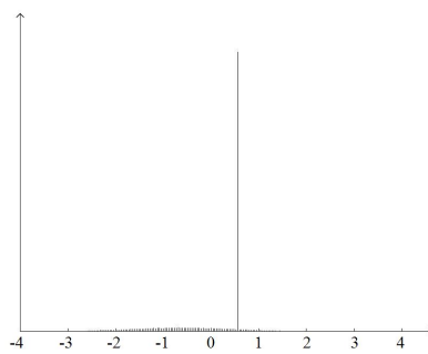
(F.b) \Delta(0, 1, -\frac{2}{\sqrt{3}}, \frac{10}{9})
