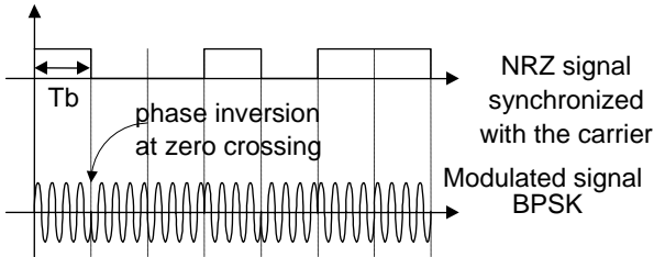
Fig 3 : Modulation BPSK
