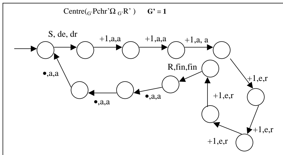
Figure 9: automata de décision
