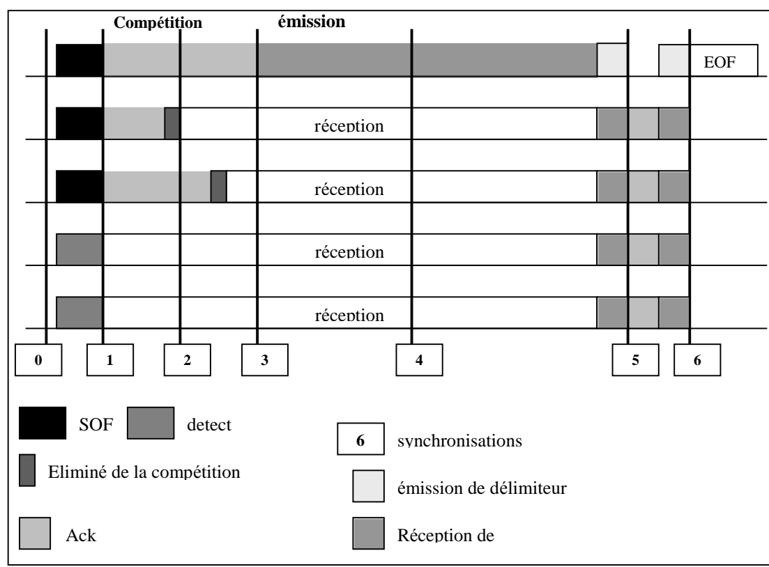
Figure 12 : exemple d'exécution simultanée de drivers
