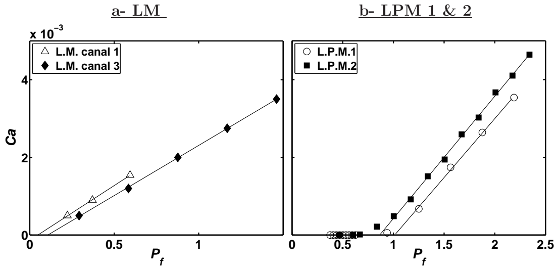
FIG. 2.13: Courbes Ca - P_f pour L_{ad} = 100 . a- Liquide mouillant pour deux géométries (Canal 1 & 3). b- Liquides partiellement mouillants (Canal 2). Les droites sont des régressions des points expérimentaux (obtenues pour P_f > 1 pour les LPM).
