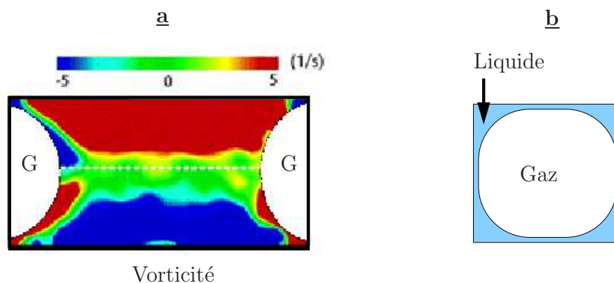
FIG. 1.3: Quelques caract ristiques de l' coulement de bouchons dans un microcanal de section carr e (G nther et al. , 2005). a- Des zones de recirculation existent dans le bouchon. En mesurant par P.I.V. (Particle Image Velocimetry) le champ des vecteurs vitesse dans le bouchon en  coulement, les auteurs ont mesur  la vorticit , qui est notamment importante dans les r gions confin es entre les interfaces et les parois du canal. b- Le sch ma illustre la pr sence de liquide, autour des bulles de gaz et dans les coins du microcanal.
