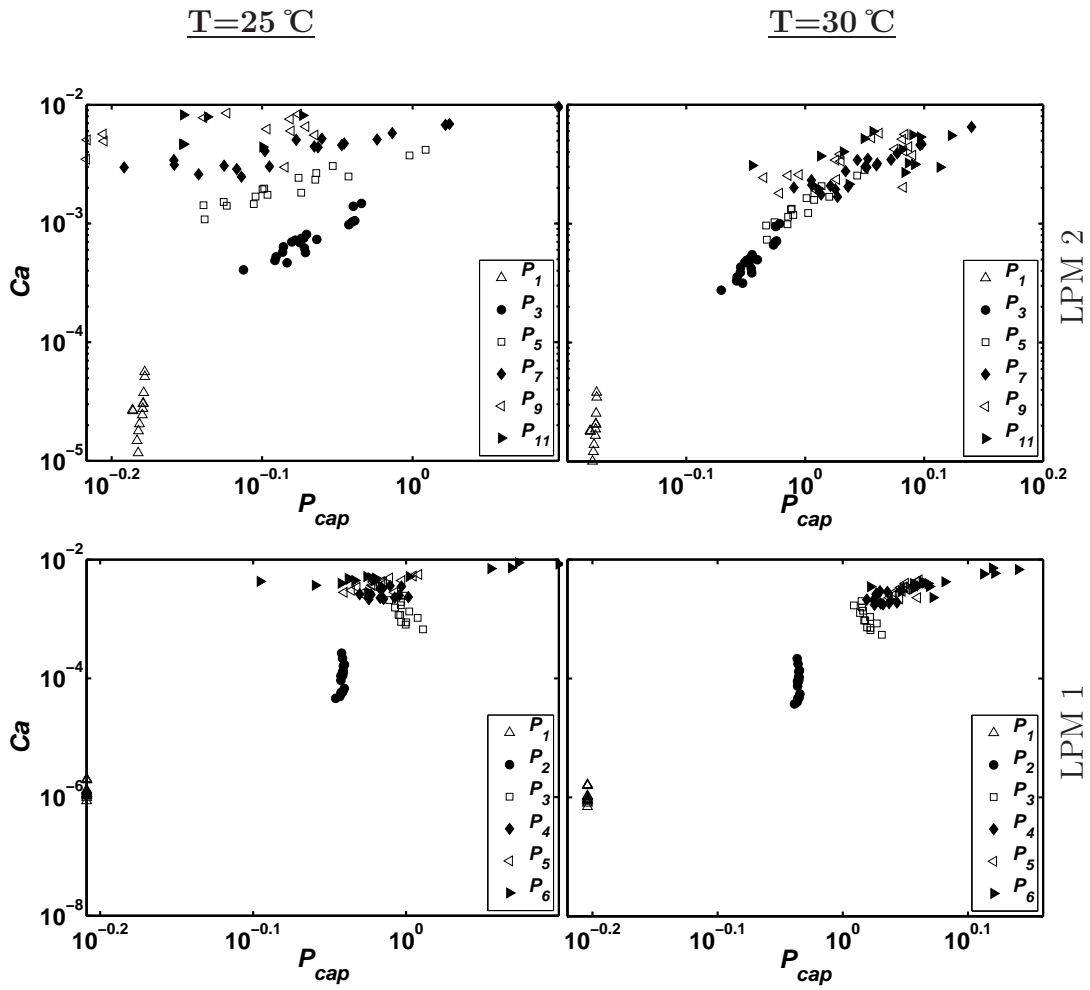
FIG. B.1: Termes capillaires pour les liquides partiellement mouillants, obtenus pour deux températures différentes : à gauche T=25\text{ }^{\circ}\text{C} , à droite T=30\text{ }^{\circ}\text{C} . Les graphiques du dessus correspondent à la solution aqueuse de glycérol (LPM 2), et ceux du dessous à l'eau (LPM 1). Les pressions sont les mêmes que celles des courbes de la figure 2.11.
