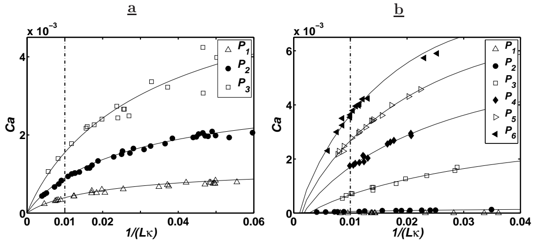
FIG. 2.12: Courbes Ca - (L\kappa)^{-1} (Vitesse adimensionnée-Inverse de la longueur adimensionnée). a- Le liquide mouillant b- Le LPM 1. Les courbes en trait continu qui approchent les points expérimentaux sont obtenues par des régressions aux moindres carrés non linéaires. Elles permettent l'interpolation des nombres capillaires aux différentes pressions de forçage pour une longueur adimensionnelle L_{ad} = 100 .
