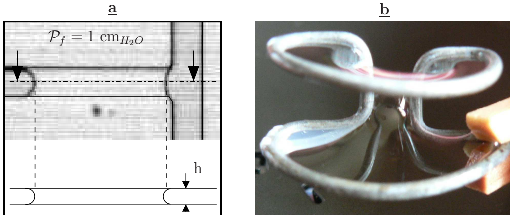
FIG. 4.1: a- Vues de dessus et de côté des bouchons en situation de blocage. b- Montage permettant de se faire une idée de la forme de l'interface avant du bouchon en blocage, en vue de face, c'est à dire, sortant du microcanal.
