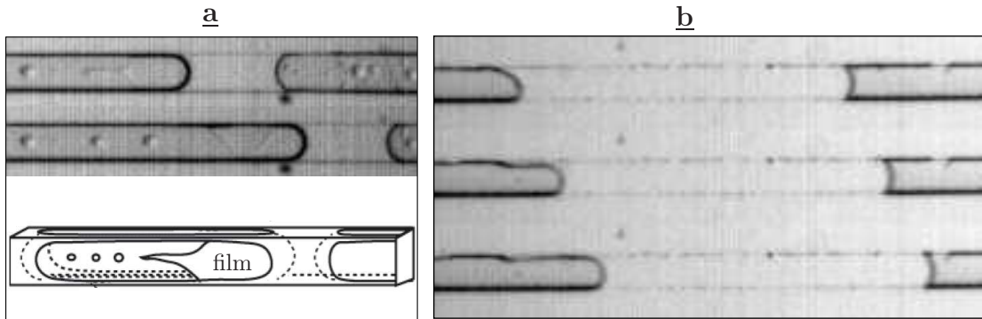
FIG. 2.16: Quelques observations pour des bouchons se déplaçant à des vitesses élevées ( Ca \simeq 5 \cdot 10^{-3} ). a- On observe après le passage du bouchon des parois plus sombres, synonymes du dépôt d'un film liquide à l'interface arrière. Ce film est ensuite déstabilisé par une ligne de contact, et le liquide démouille pour former des gouttes dans le microcanal. Le schéma, issu de (Jensen et al. , 2004), illustre ce phénomène. b- A grande vitesse, l'accrochage de la ligne de contact des bouchons de liquide partiellement mouillant provoque le dépôt d'un film.
