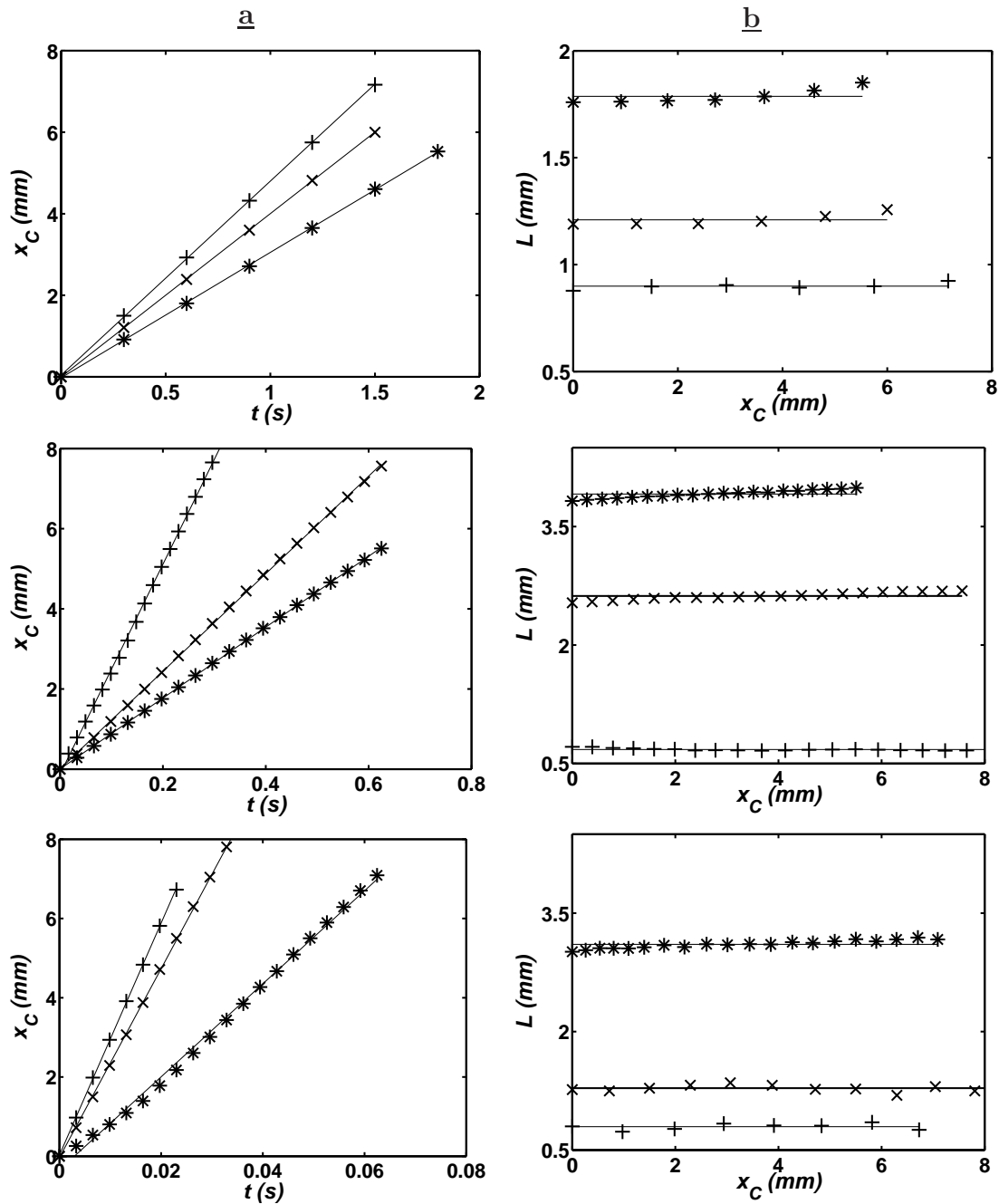
FIG. 2.9: a- Positions successives du centre du bouchon en fonction du temps. Trois bouchons de longueur différente sont considérés sur chaque graphe. Les droites sont des régressions linéaires des points expérimentaux. b- Evolution des longueurs correspondantes lors du trajet des bouchons. Les droites correspondent aux longueurs moyennes. De haut en bas , LM ( P_f = 2.5 \text{ cm}_{H_2O} ), LPM 2 ( P_f = 30 \text{ cm}_{H_2O} ), LPM 1 (eau, P_f = 50 \text{ cm}_{H_2O} ).
