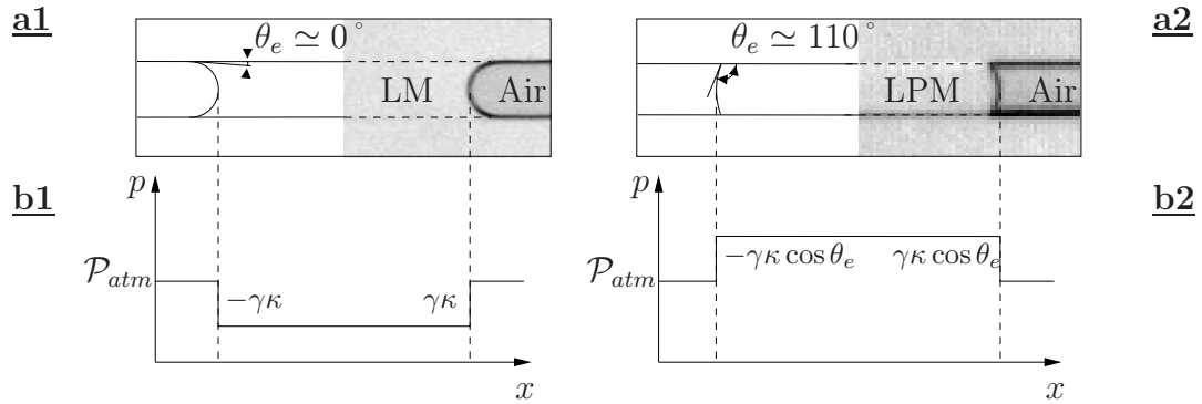
FIG. 2.3: Les figures du haut (a) sont des photos obtenues à l'aide d'un microscope et des schémas de bouchons de liquides mouillant (LM, a1) et partiellement mouillant (LPM, a2) au repos dans un microcanal. Elles montrent la forme des interfaces dans les deux cas, ainsi que les angles de contact. Pour le LM, l'angle de contact \theta_e est proche de 0^\circ tandis qu'il est supérieur à 90^\circ pour le LPM. Les figures du bas (b) montrent la pression p dans le canal en fonction de la position x . Les courbures moyennes des interfaces (respectivement \kappa = 2/h + 2/w pour le LM et \kappa \cos \theta_e pour le LPM) permettent de calculer les sauts de pression aux interfaces par la loi de Laplace. Le LPM est en surpression (b2) tandis que le LM est en dépression (b1) par rapport à l'air à pression ambiante \mathcal{P}_{atm} .
