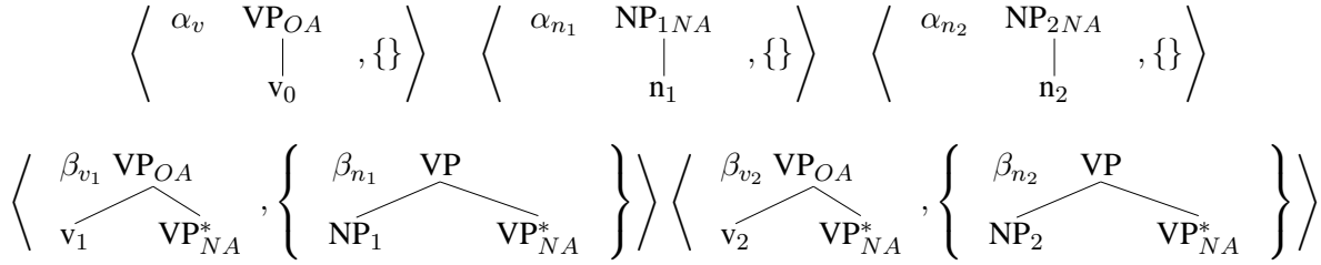
FIG. 4 – TT-MCTAG
