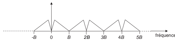
Fig. 4.3 Densité spectrale de puissance d'un signal en bande passante (cas N impair) échantillonné à 2B
