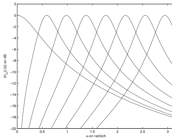
Fig. D.1 Module des fonctions de transfert des filtres du banc d'analyse « Banc1 »
