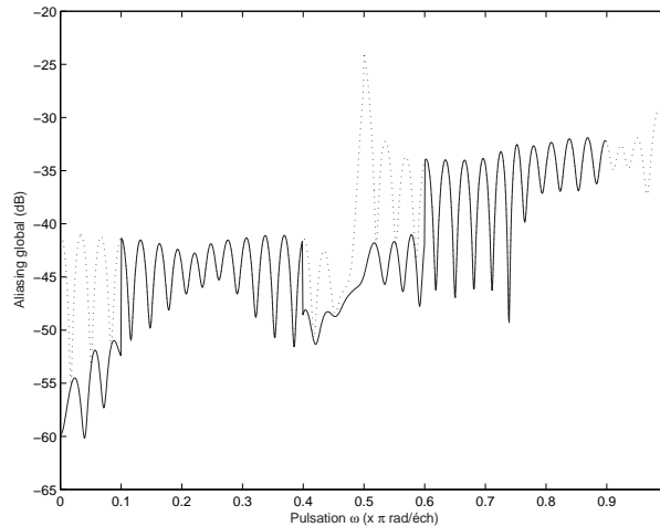
Fig. 3.22 Repliement total - méthode AC et paramètres du tableau 3.13. En trait pointillé : \eta_X = 1 . En trait plein : \eta_X = 0.9
