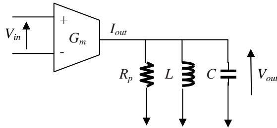
Fig. 3.1 Résonateur Gm-LC
