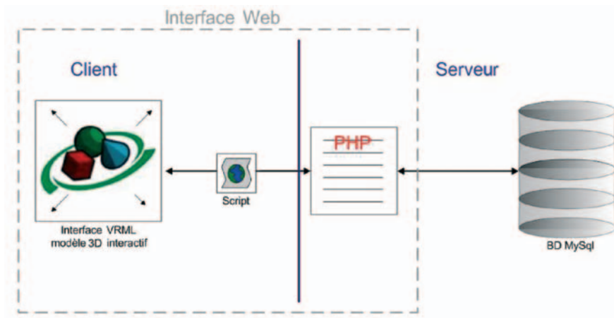
Figure 6. Fonctionnement informatique du système d'information (d'après Meyer et al., 2006)
