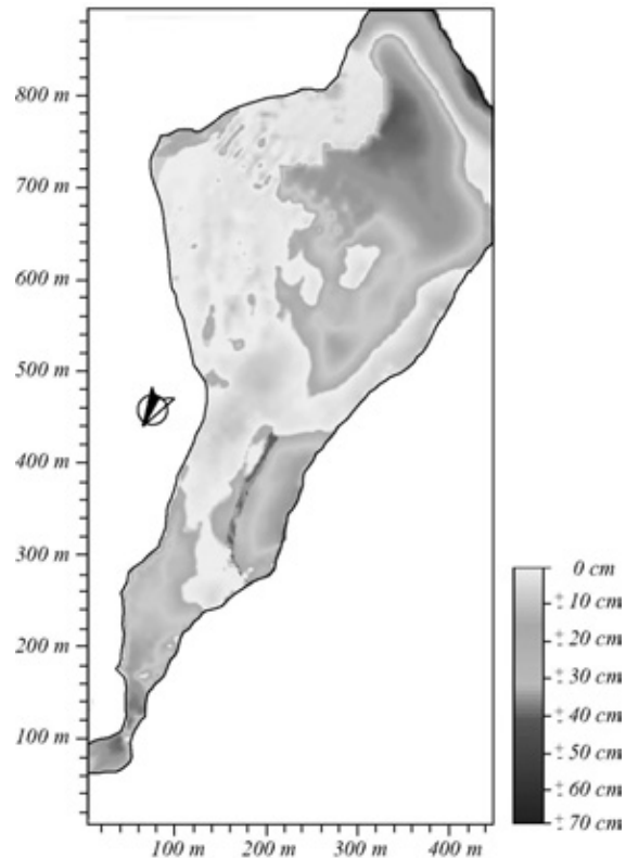
Figure 5. Carte des différences entre MNT photogramétrique et tachéométrique
