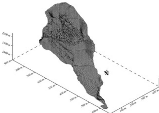
Figure 4. Représentation du MNT obtenu par voie photogramétrique
