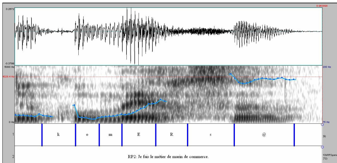
Figure 3: Exemple d'un plateau haut réalisé sur une syllabe atone (avec schwa), logiciel PRAAT, transcription phonétique du mot commerce en SAMPA
