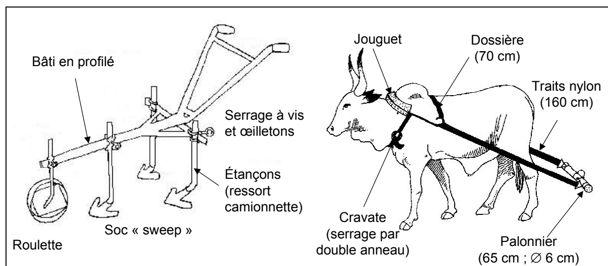
Figure 7. Schémas de la houe Attila et de du jouguet monobovine IRAD BF.
