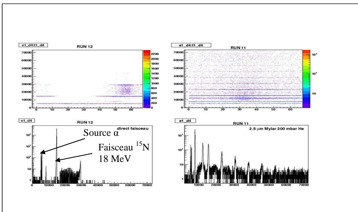
Figure II-20 Dans la partie gauche sont présentés : le spectre énergie versus temps de vol (en haut) et le spectre énergie (en bas) obtenus sans cible gazeuse (faisceau directement sur le détecteur). On observe des événements de pile up. Dans la partie droite sont présentés les mêmes spectres obtenus avec la cible gazeuse placée dans la ligne de faisceau. Dans cette partie nous observons une multitudes de pics d'énergies inattendues qui correspondent à des événements qui déposent dans notre détecteur une énergie (très) supérieure à celle du faisceau incident !
