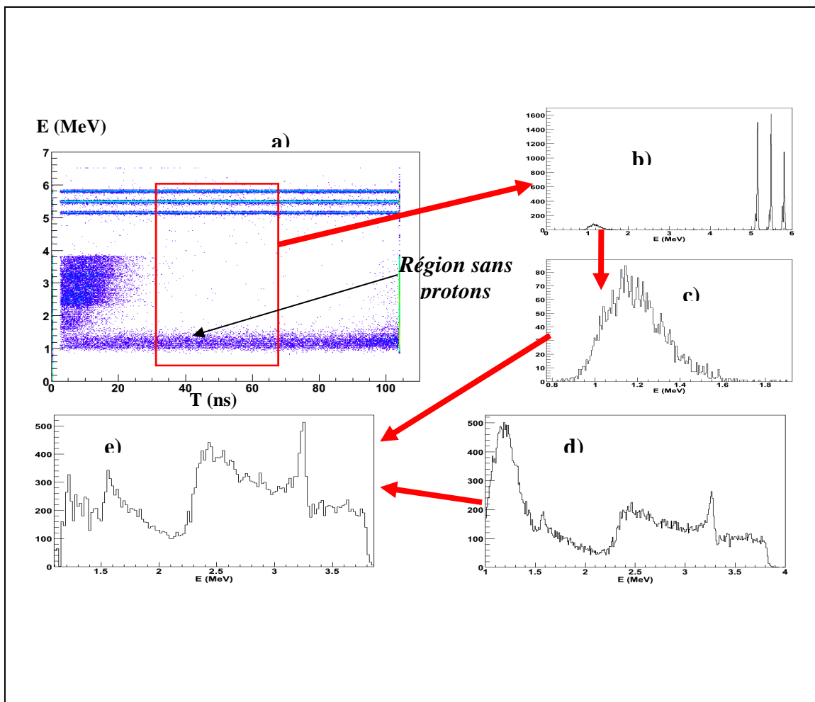
Figure III-7 Présentation schématique de la méthode utilisée pour éliminer le bruit de fond bêta. Cette méthode a été utilisée pour obtenir la fonction d'excitation {}^1\text{H}({}^{15}\text{O},\text{p}){}^{15}\text{O} . A partir de l'image bidimensionnelle énergie versus temps de vol (a), nous sélectionnons une région dans laquelle il n'y a pas des protons dans le bruit de fond bêta (la région encadrée). Nous faisons la projection sur l'axe Y (énergie) des événements qui se trouvent dans cette région. Ainsi nous obtenons le spectre b). Dans la partie des hautes énergies, nous retrouvons les particules \alpha en provenance de la source trois pics alpha. A basse énergie, nous n'avons que le bruit de fond bêta. Ce bruit de fond est mieux montré dans le spectre c). Maintenant, nous connaissons la dépendance avec l'énergie du bruit de fond bêta. Mais, pour extraire ce fond du spectre d) correspondant aux protons, il faut connaître le nombre total de bêtas dans ce spectre. Parce que le temps de demi-vie pour les noyaux radioactifs d' {}^{15}\text{O} est de 2.03 m, et parce que toute l'échelle de notre mesure de temps de vol est 100.47 ns, il n'y a pas de corrélation entre le « start » de la mesure de temps donné par le positron et le « stop » de la mesure donné par la haute fréquence de cyclotron. Dans ce cas, les événements bêtas sont uniformément distribués sur l'axe de temps de vol. C'est la même situation que nous retrouvons pour les particules \alpha . La source alpha est complètement décorrélée par rapport à la fréquence HF du cyclotron. Dans ce cas, le rapport entre les particules \alpha et les bêtas dans le spectre b) est identique avec le rapport dans spectre total a). C'est ainsi que nous avons une normalisation du bruit de fond bêta.
