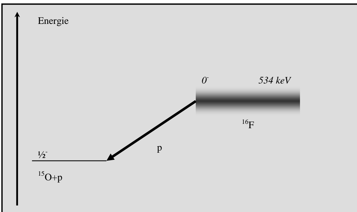
Figure I-3 Le niveau fondamental du ^{16}\text{F} est au dessus du seuil d'émission proton par 534 keV. La largeur considérée (voir référence [Til93] de ce niveau fondamental est de 40 \pm 20 keV. A cause de sa largeur, le niveau fondamental de ^{16}\text{F} a un temps de vie très court ( \sim 1.2 \cdot 10^{-20} s). Il décroît vers l'état fondamental d' ^{15}\text{O} .
