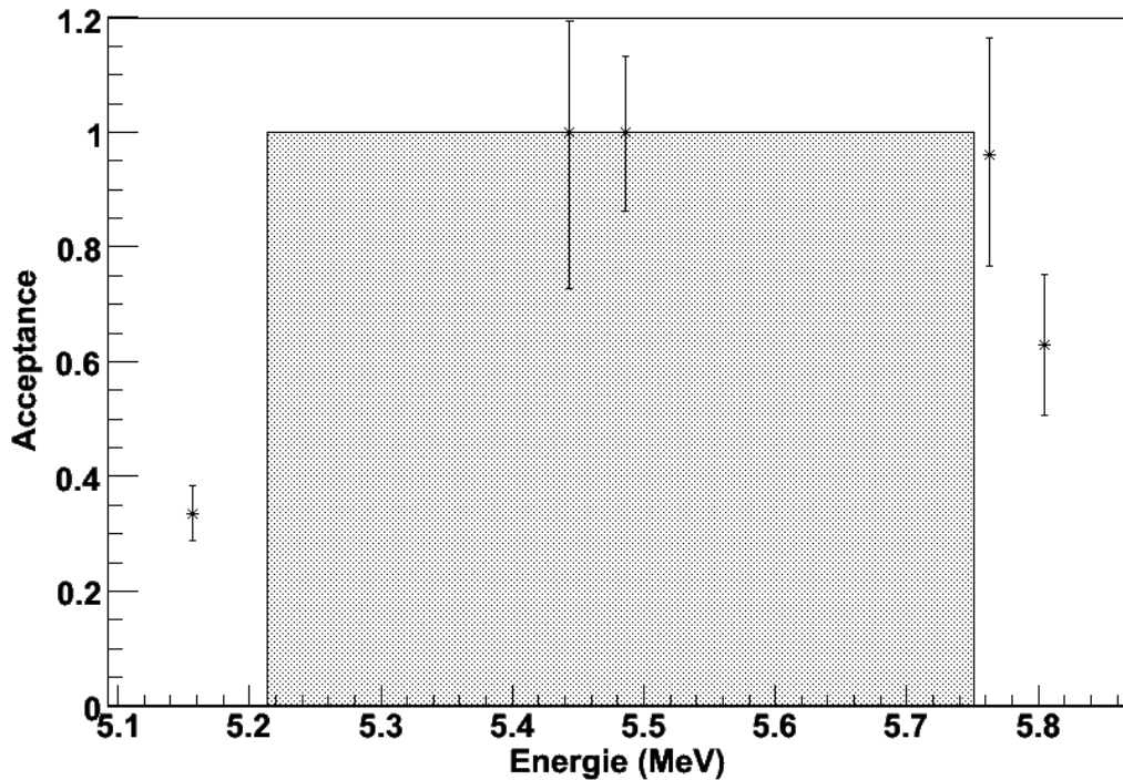
Figure II-15 Mesure de l'acceptance de LISE pour une rigidité magnétique 0.337 Tm. La zone grisée est la région où nous attendons une acceptation de 100 %.
