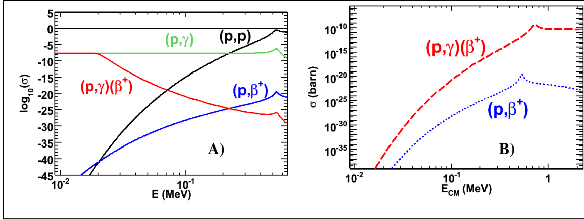
Figure III-22 Section efficace de la réaction ^{15}\text{O}(p,\gamma)(\beta^+)^{16}\text{O} , et comparaison avec la section efficace de la réaction ^{15}\text{O}(p,\beta^+) . Dans la figure A), nous avons représenté différents termes de l'équation III-20, et la comparaison avec les réactions ^{15}\text{O}(p,p)^{15}\text{O} et ^{15}\text{O}(p,\beta^+) . La courbe (p,γ) représente la section efficace de la réaction ^{15}\text{O}(p,\gamma)^{16}\text{F}^{\text{gs}} de peupler l'état fondamental de ^{16}\text{F} à une énergie relative E entre le proton et ^{15}\text{O} (calculé pour une énergie dans le système de centre de masse égale à 0.729 MeV). La courbe (p,γ)(β + ) représente la section efficace de la réaction ^{15}\text{O}(p,\gamma)(\beta^+)^{16}\text{O} peuplant l'état fondamental de ^{16}\text{F} (peuplé par la transition gamma) à une énergie finale relative E entre le proton et l' ^{15}\text{O} (la courbe est calculée pour une énergie incidente proton égale à 0.729 MeV). Dans la figure B, nous avons représenté la dépendance avec l'énergie dans le système de centre de masse de la section efficace de réaction (p,γ)(β + ) et la comparaison avec la section efficace de réaction (p,β + ) calculé auparavant.
