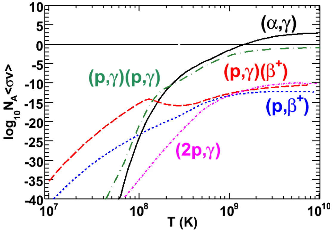
Figure III-27 Le calcul de taux ( fait avec le code numérique PNINR) pour la réaction ^{15}\text{O}(p,\gamma)(p,\gamma)^{17}\text{Ne} et la comparaison avec les autres processus possibles à partir d' ^{15}\text{O} - ^{15}\text{O}(2p,\gamma)^{17}\text{Ne} , ^{15}\text{O}(\alpha,\gamma)^{19}\text{Ne} , ^{15}\text{O}(p,\beta^+)^{16}\text{O} et ^{15}\text{O}(p,\gamma)(\beta^+)^{16}\text{O} . Les deux taux de réactions, (p,\gamma)(\beta^+) et (p,\gamma)(p,\gamma) , sont limités par la probabilité de capture radiative ^{15}\text{O}(p,\gamma)^{16}\text{F}^{\text{gs}} . Pour la réaction (p,\gamma)(p,\gamma) , la densité du milieu astrophysique utilisé pour le calcul est de 10^6 \text{ g/cm}^3 .
