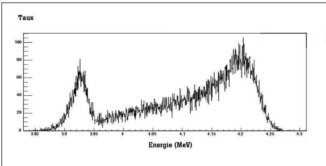
Figure II-19 Fonction d'excitation attendue pour la réaction {}^4\text{He}({}^{15}\text{N},\alpha){}^{15}\text{N} . Le calcul a été fait avec la théorie de la matrice R à partir des états connus du noyau composé pour cette réaction, le {}^{19}\text{F} .
