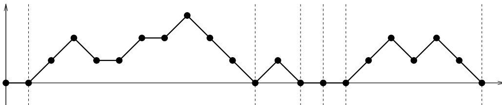
Un chemin de Motzkin de longueur 21 et ses 6 facteurs premiers.
