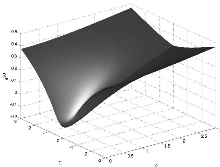
FIG. 5.1: Fonction métrique e^{2U} pour m = 1 , \phi = \frac{\pi}{4} et \delta = 4.1 .
