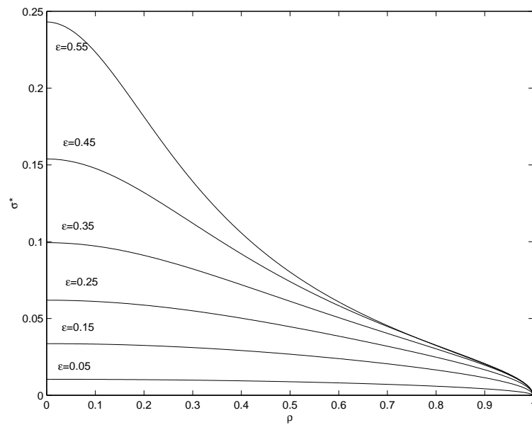
FIG. 4.13: Densité d'énergie \sigma^* pour \gamma = 0.7 et plusieurs valeurs de \epsilon .
