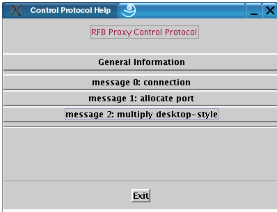
FIG. E.4 – La fenêtre principale d'aide offerte par l'interface graphique du contrôleur à distance.
