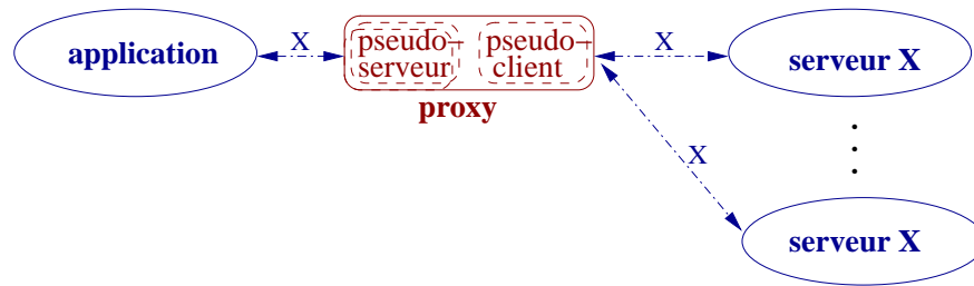
FIG. 2.10 – Architecture centralisée. Un proxy est interposé entre le client et le serveur X. Il est vu comme un serveur habituel par l'application et comme un client X par les serveurs.
