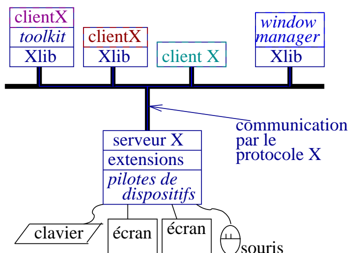
FIG. 2.9 – Structure du système X (dessin adapté du [57]). Les applications et le serveur X peuvent se trouver sur la même machines ou sur des machines différentes.
