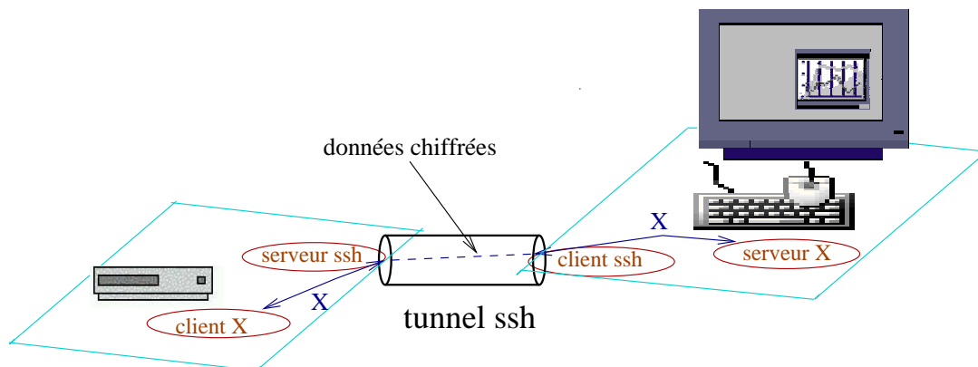
FIG. 2.8 – Acheminement d'une session X par ssh.
