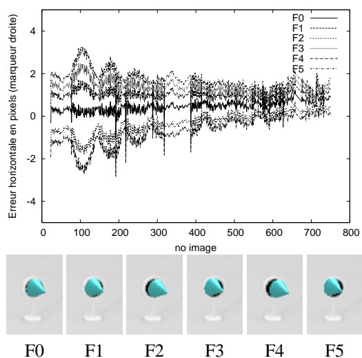
FIG. 9 – Influence de la distance focale sur l’alignement 2D.
