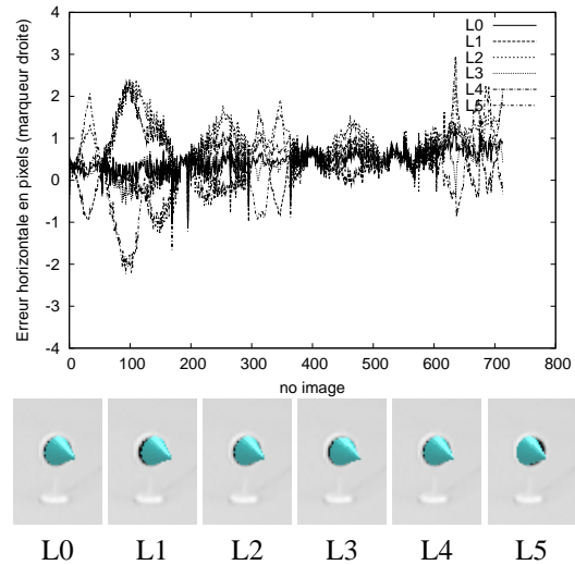
FIG. 10 – Influence des paramètres de distorsion sur l’alignement 2D.
