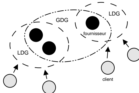
Figure 1: Architecture hiérarchique de JuxMem.
