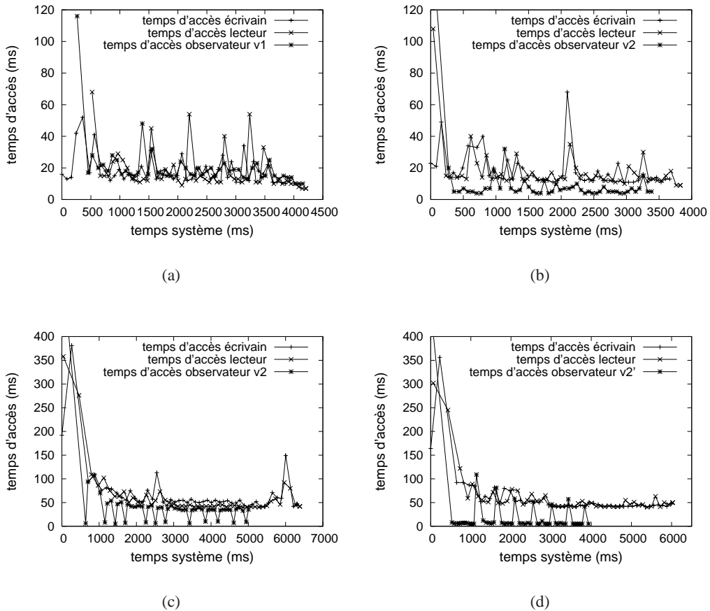
Figure 2: Temps d'accès à une donnée partagée. (a) v_1 , 1 ko. (b) v_2 , 1ko, D = 0 , w = 0 . (c) v_2 , 1024 ko, D = 0 , w = 0 . (d) v'_2 , 1024 ko, D = 3 , w = 6 .
