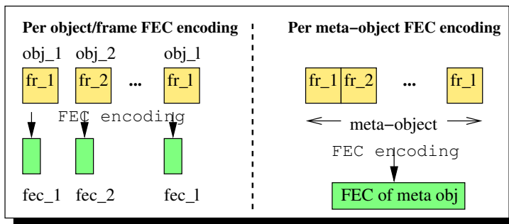
Figure 11.1: Per object versus per meta-object FEC encoding.
