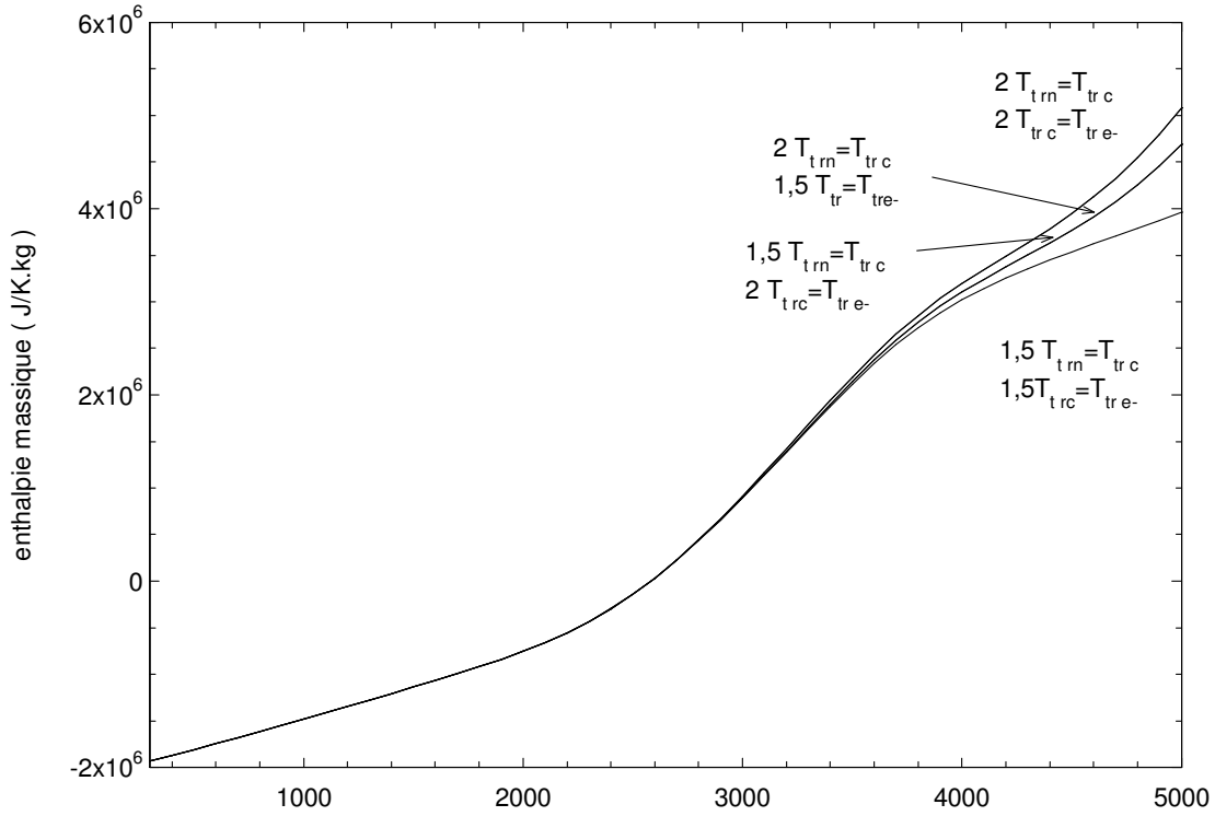
Figure II.29 :Enthalpie massique d'un plasma Ar-CO 2 (Ar 80%, 20% CO 2 ) pour différents déséquilibres de températures en fonction de la température des espèces neutres T_{rn} (K).
