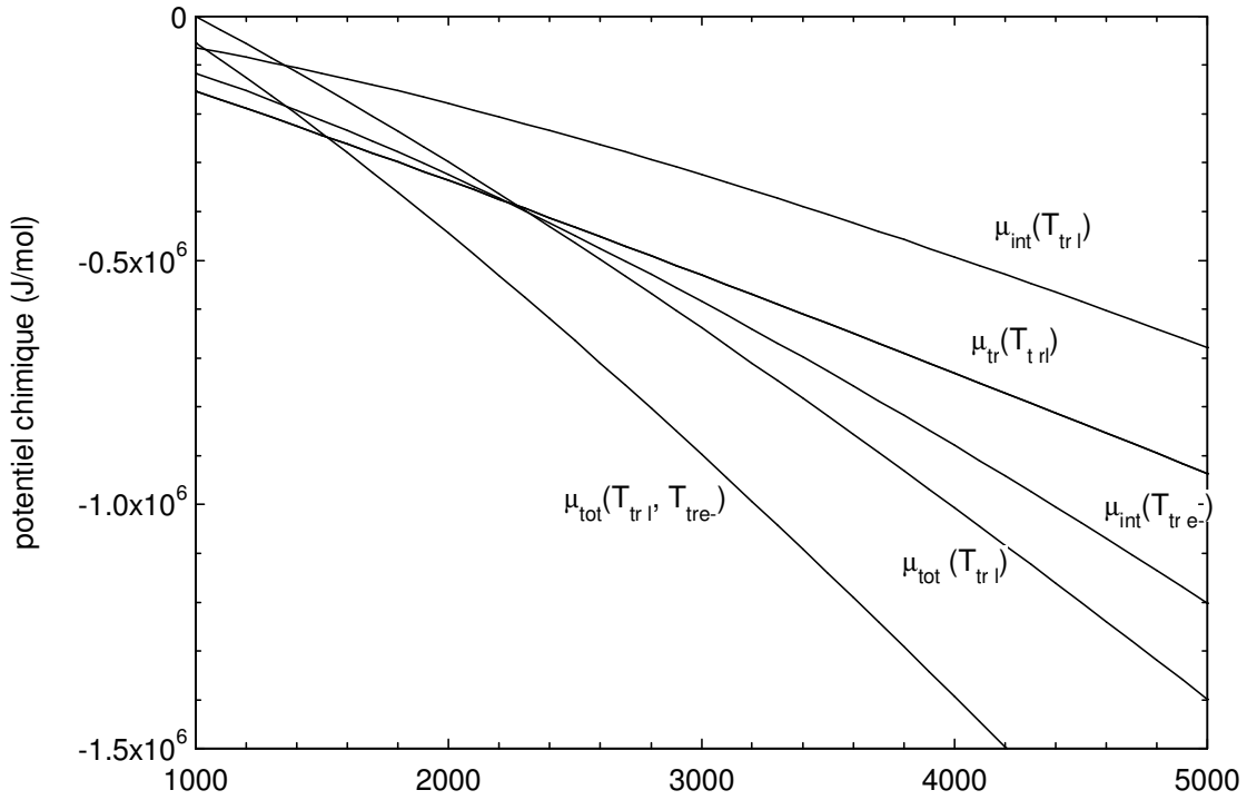
Figure II.16 : Potentiels chimiques de translation, interne et total de la molécule d'éthine C 2 H 2 dans un plasma de polyéthylène ( T_{\text{tr } e^-} = 1,5 T_{\text{tr } l} ).
