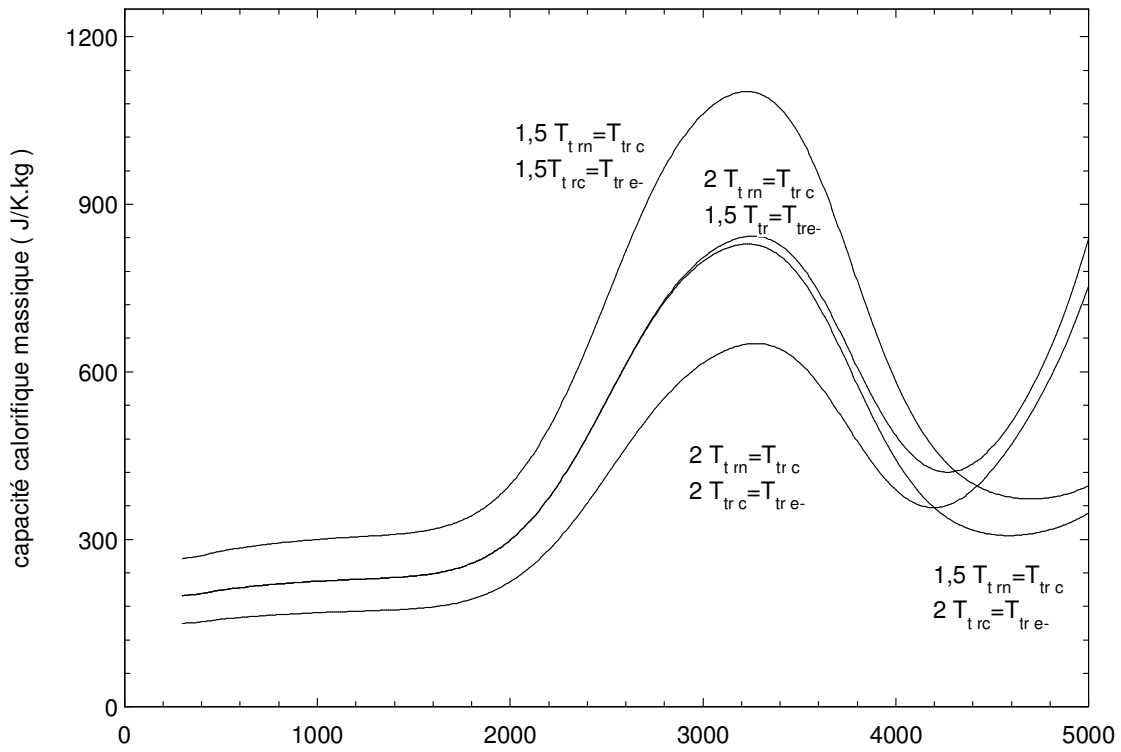
Figure II.30 :Capacité calorifique massique d'un plasma Ar-CO 2 (Ar 80%, 20% CO 2 ) pour différents déséquilibres de températures en fonction de la température des espèces neutres T_{rn} (K).
