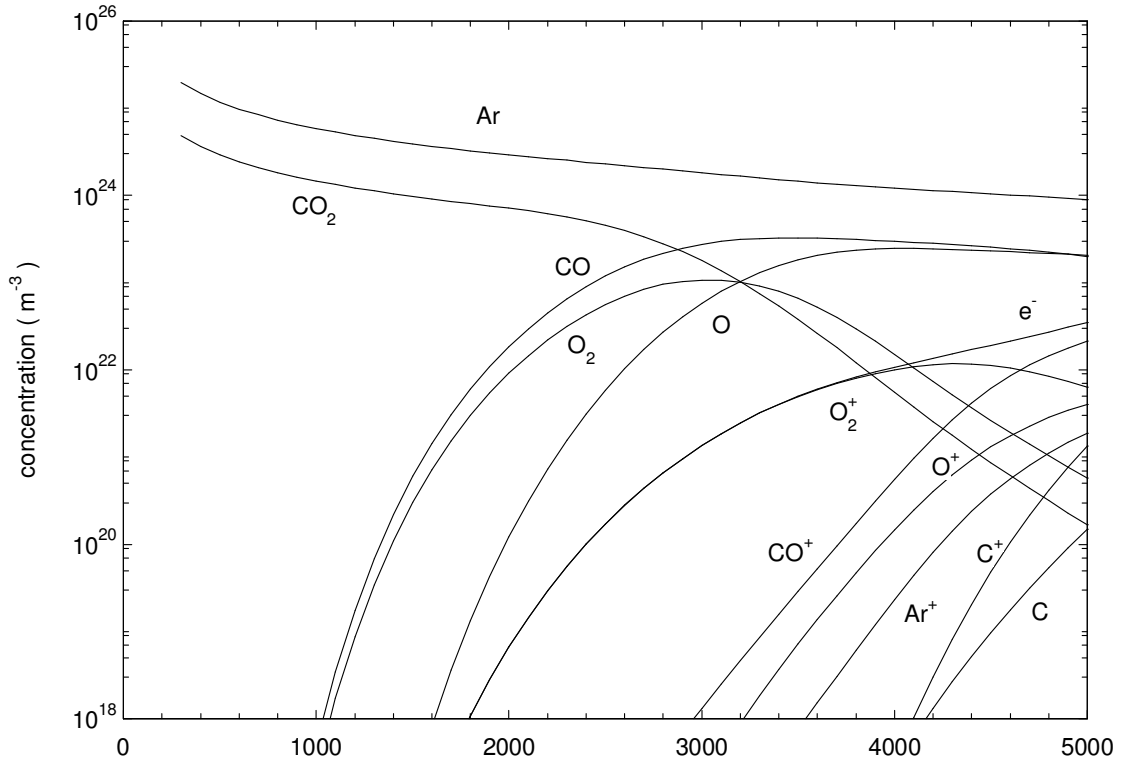
Figure II.26 : Composition d'un mélange Ar-CO 2 (Ar 80%, 20% CO 2 ) pour le déséquilibre : 2T_{trn} = 2T_{trc} = T_{tr e-} en fonction de la température des espèces neutres T_{trn} (K).
