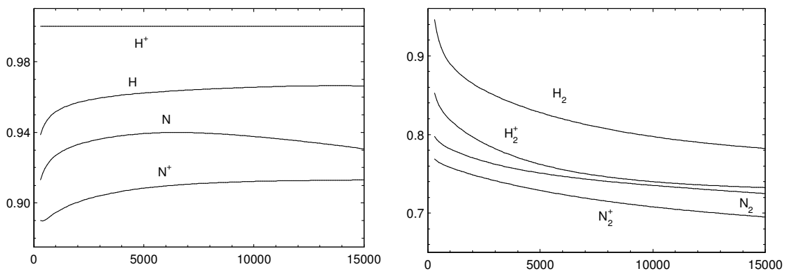
Figure II.9 : Rapport \frac{\mu_{tr}}{\mu_{tot} - e^0} des plasmas d'azote et d'hydrogène en fonction de la température (K) à l'équilibre thermique.
