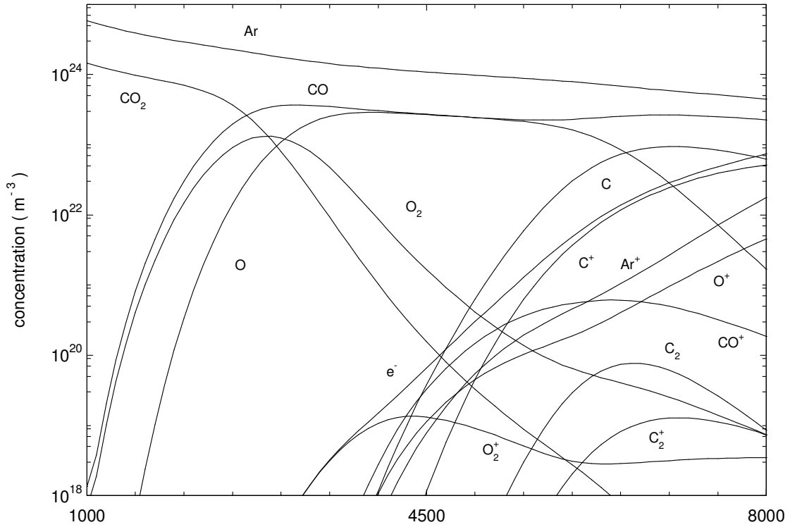
Figure II.20 : Composition d'un mélange argon \text{CO}_2 (Ar 80%, 20% \text{CO}_2 ) pour un déséquilibre \theta = 1,5 à la pression atmosphérique en fonction de la température des espèces lourdes (K).
