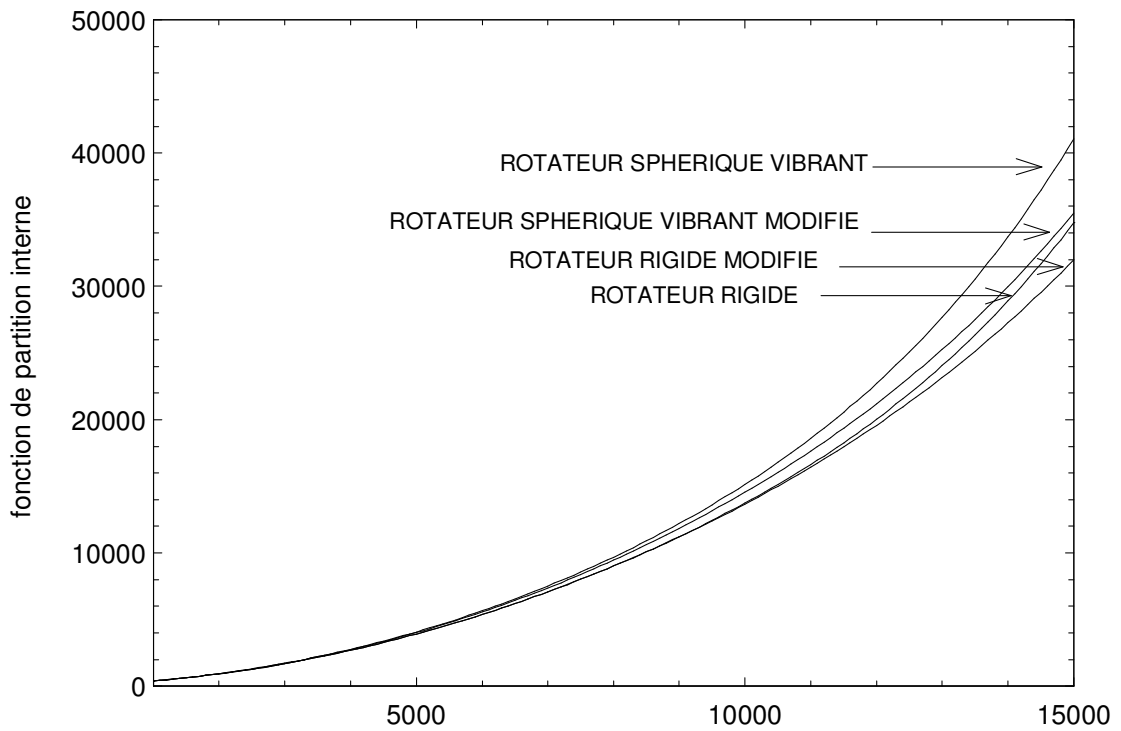
Figure II.4 : Comparaison des résultats obtenus par les différentes méthodes de calculs de la fonction de partition interne (eq. II.48, II.49, II.53 , II.54 ) de CO.
