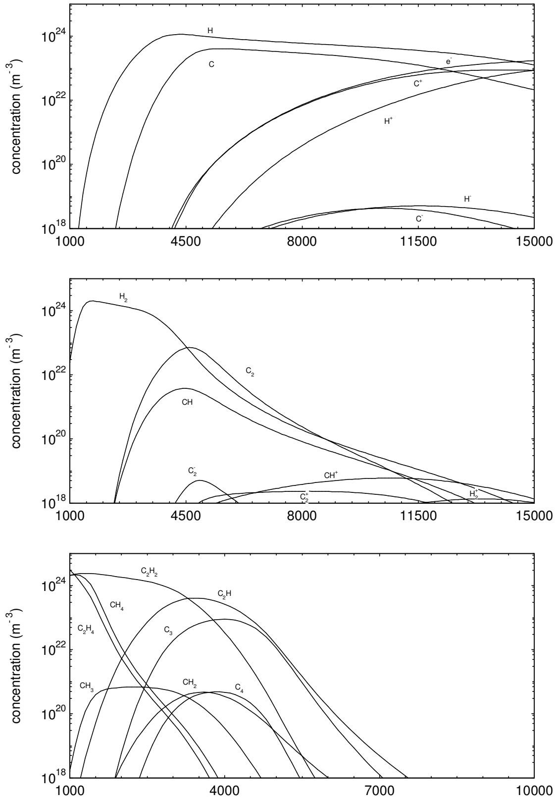
Figure I.15 : Evolution de la concentration des espèces monoatomiques, diatomiques et polyatomiques en fonction de la température (K) à la pression atmosphérique du plasma de PE ( \text{CH}_2 ).
