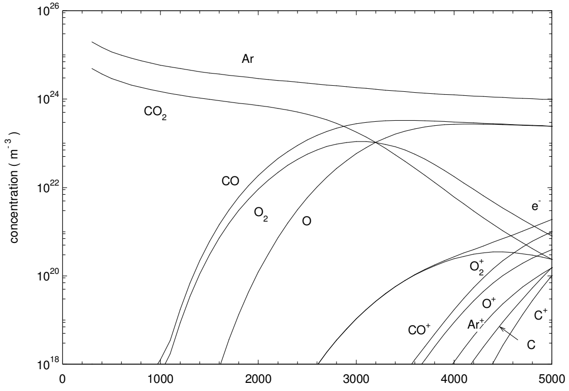
Figure II.25 : Composition d'un mélange Ar-CO 2 (Ar 80%, 20% CO 2 ) pour le déséquilibre : 1,5T_{trn} = 1,5T_{trc} = T_{tr e-} , en fonction de la température des espèces neutres T_{trn} (K).
