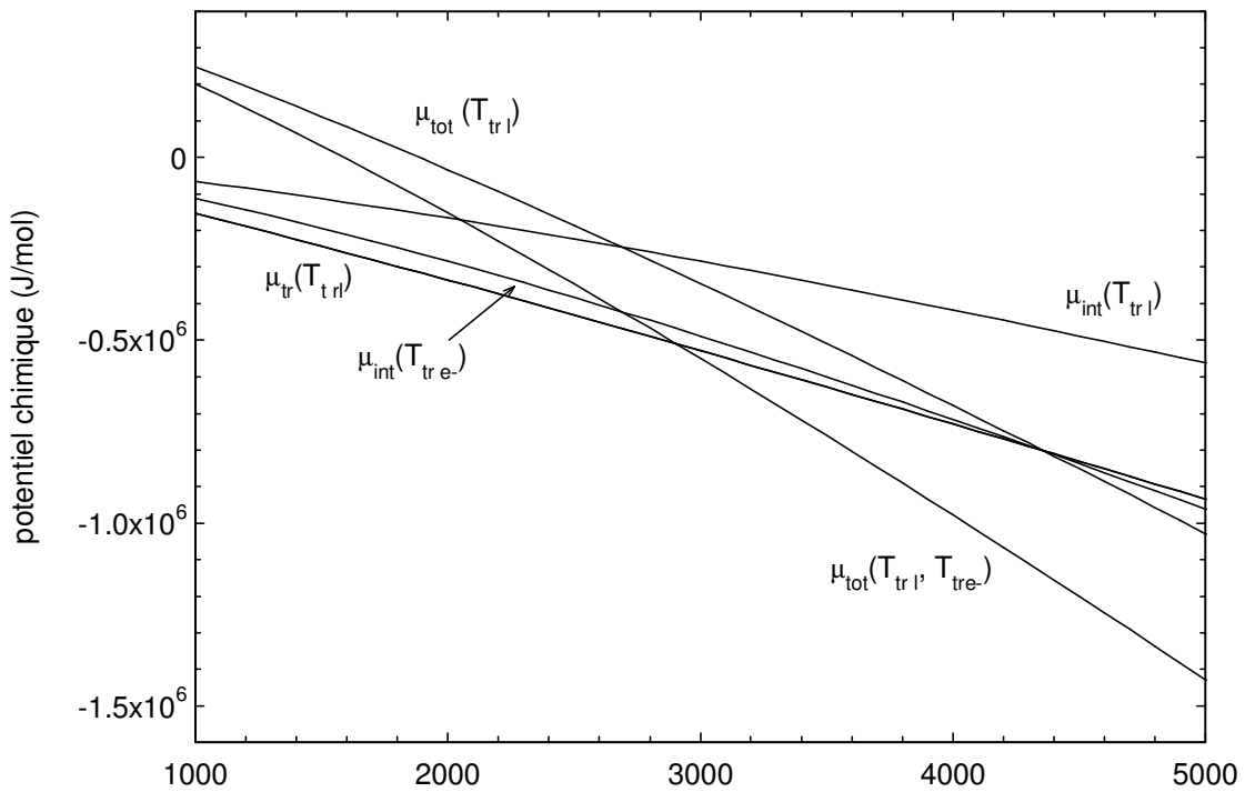
Figure II.17 : Potentiels chimiques de translation, interne et total de la molécule d'éthynyl C 2 H dans un plasma de polyéthylène ( T_{\text{tr } e^-} = 1,5 T_{\text{tr } l} ).
