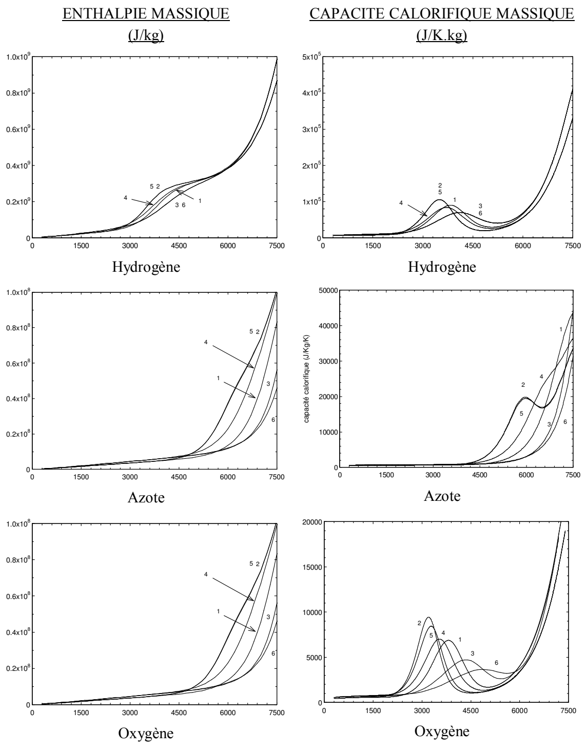
Figure II.13 : Enthalpie massique et capacité calorifique massique des plasmas d'hydrogène, d'azote et d'oxygène caractérisés par un déséquilibre \theta = 2 à la pression atmosphérique pour différentes hypothèses sur les températures internes (les chiffres correspondent aux hypothèses énoncées dans le texte)
