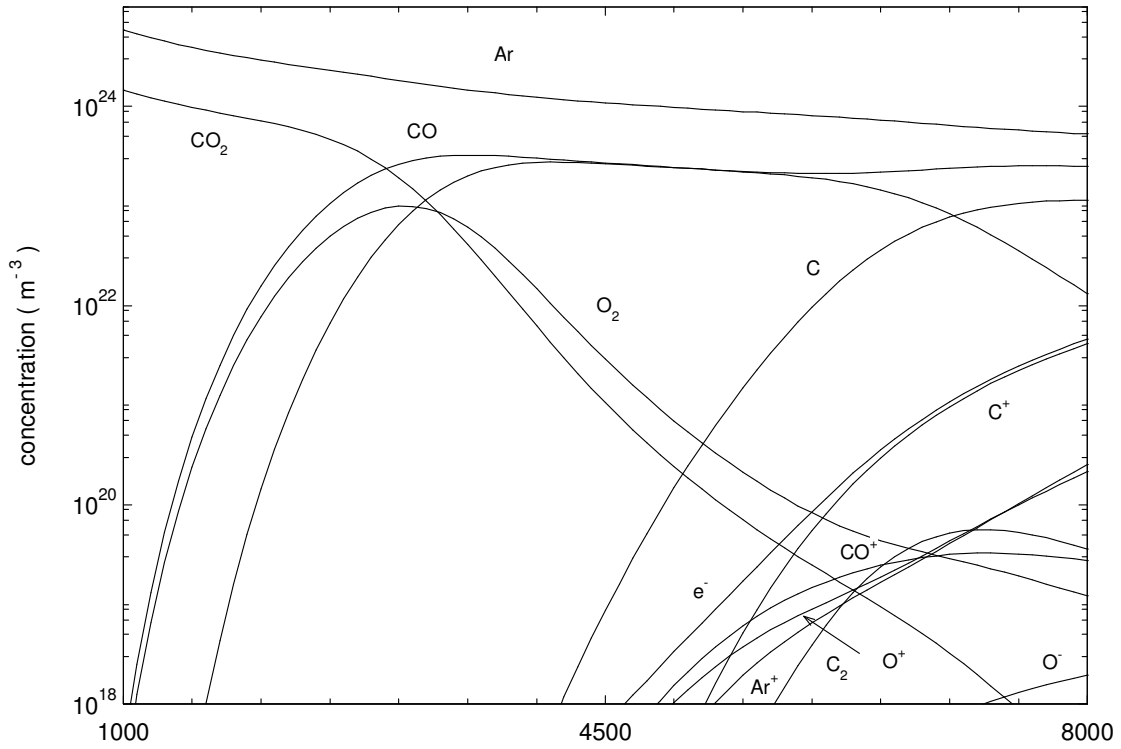
Figure II.19 : Composition d'un mélange argon \text{CO}_2 (Ar 80%, 20% \text{CO}_2 ) à l'équilibre thermique et à la pression atmosphérique en fonction de la température (K).
