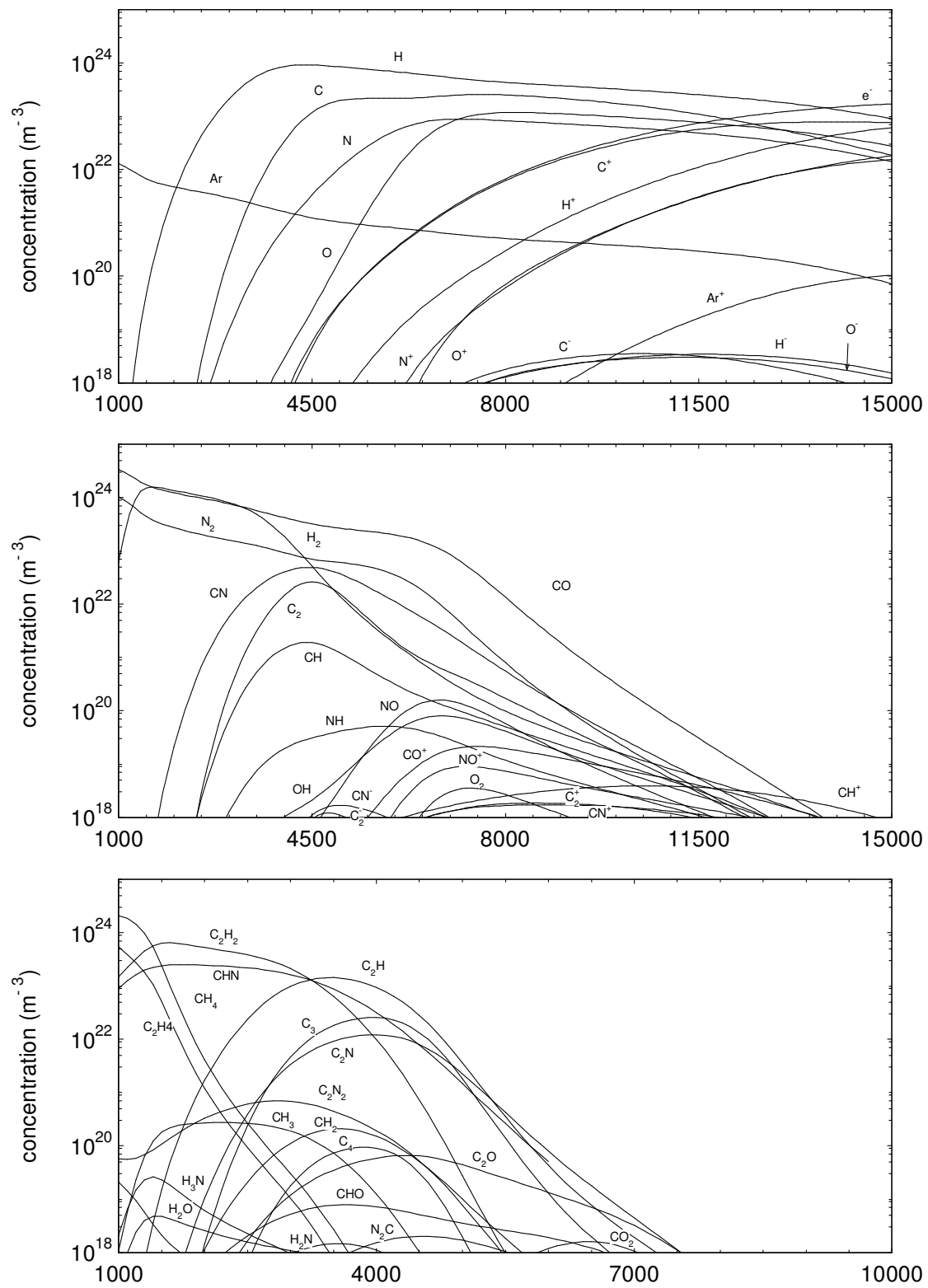
Figure I.21 : Evolution de la concentration des espèces monoatomiques, diatomiques et polyatomiques en fonction de la température (K) à la pression atmosphérique dans un mélange d'air et de PMMA (50% d'air et 50% de C 5 H 8 O 2 ).
