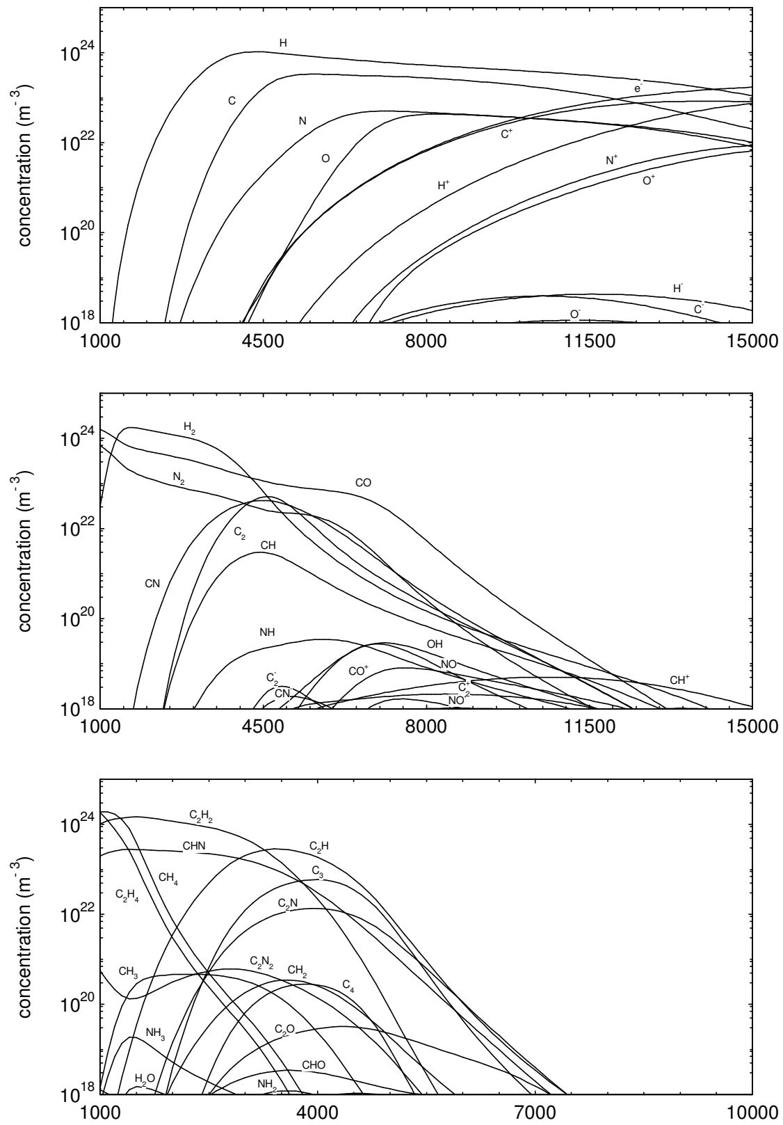
Figure I.12 : Evolution de la concentration des espèces monoatomiques, diatomiques et polyatomiques en fonction de la température (K) à la pression atmosphérique du plasma de PA 6-6 ( C_{12}H_{22}O_2N_2 ).
