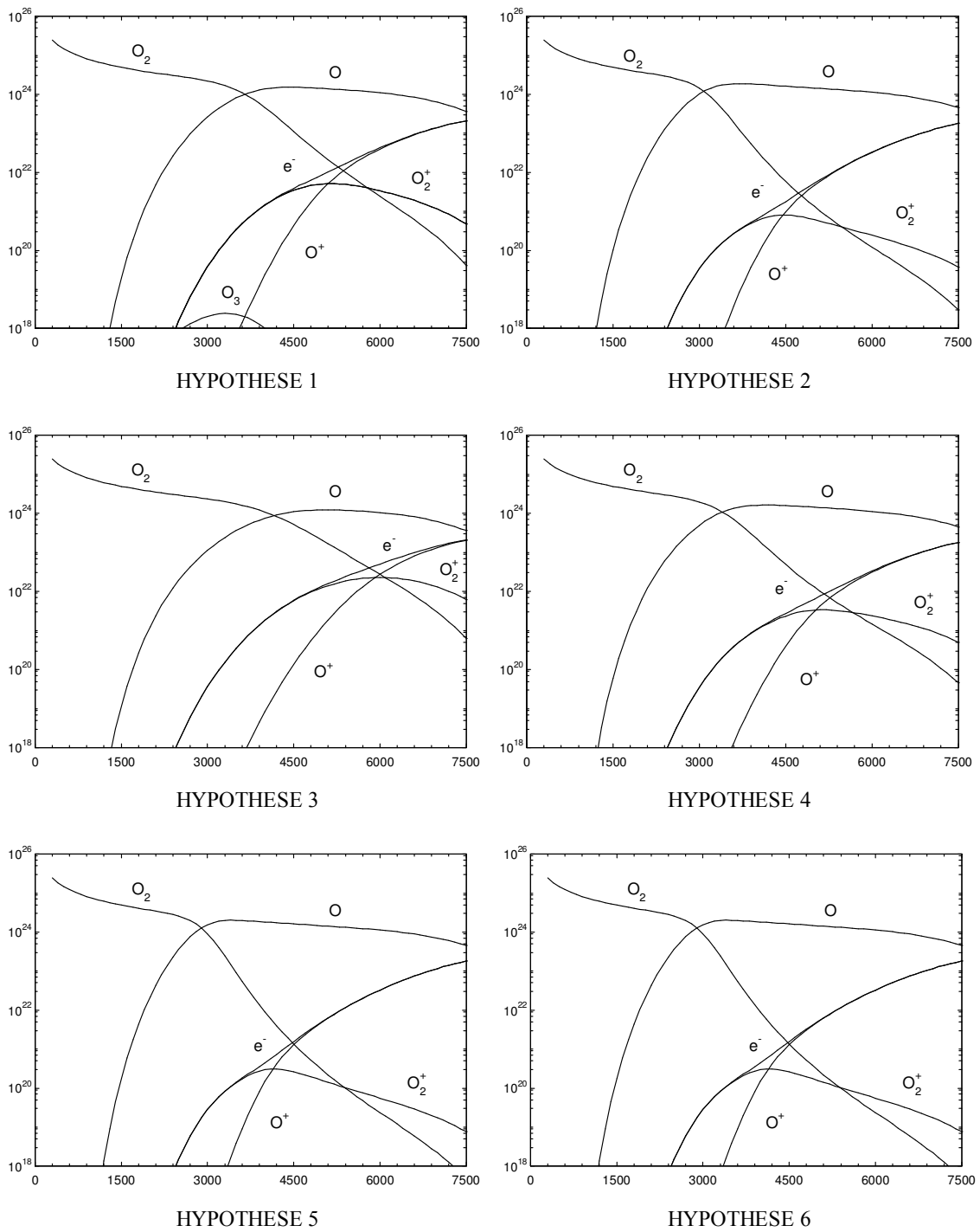
Figure II.12 : Concentration ( \text{m}^{-3} ) dans un plasma d'oxygène pur caractérisé par un déséquilibre \theta = 2 à la pression atmosphérique pour différentes hypothèses de températures. Les concentrations sont tracées en fonction de la température des espèces lourdes T_{tr,l} (K).
