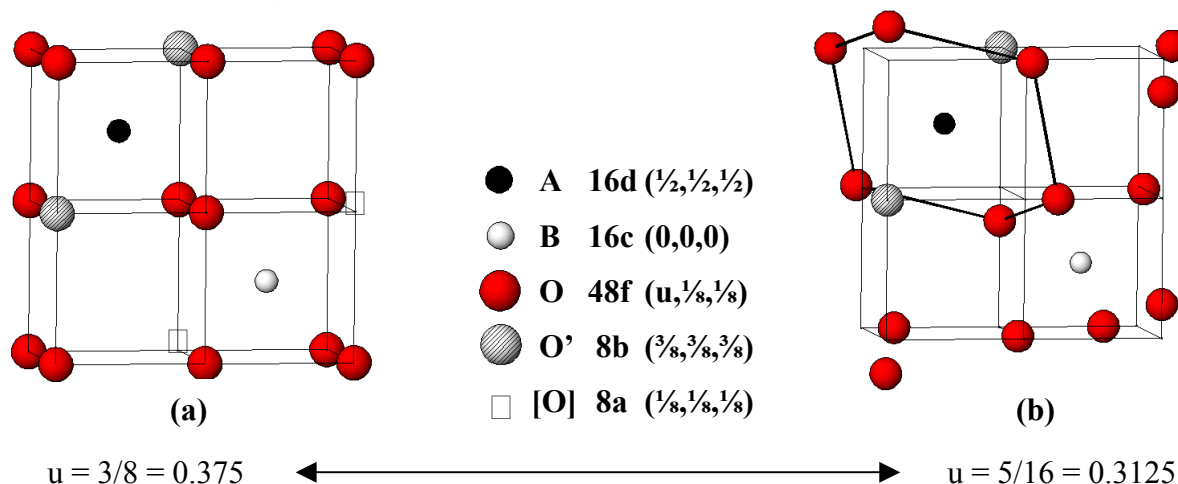
Figure I.11 : Evolution de la géométrie des sites cationiques avec la position des atomes d'oxygène en site 48f ( u, 1/8, 1/8 )
