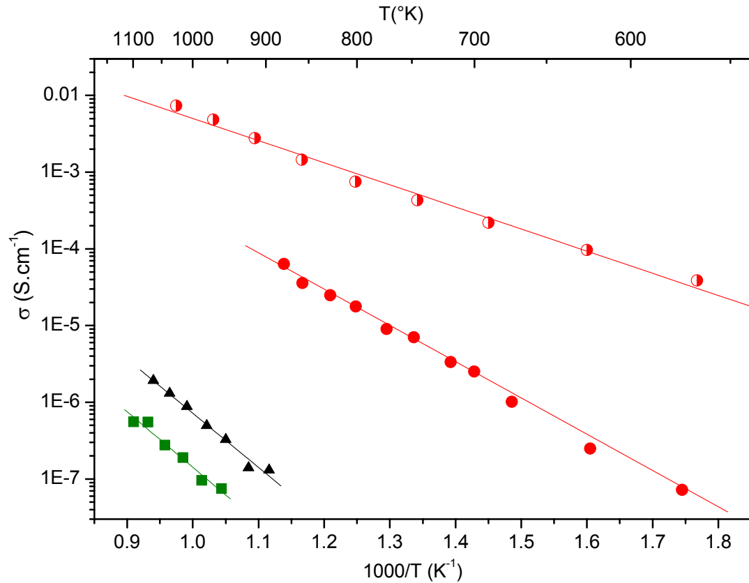
Figure IV.15 : Conductivité totale des pyrochlores Sr_{1.5}Pb_{0.2}Ga_{0.3}Ta_{1.7}O_{6.4} ( \blacktriangle ), Nd_{1.1}Pb_{0.35}Ga_{0.5}Ta_{1.5}O_{6.5} ( \blacksquare ), Ce_{1.1}Pb_{0.35}Ga_{0.5}Ta_{1.5}O_{6.84} ( \bullet ) et conductivité ionique (électrode bloquante) de Ce_{1.1}Pb_{0.35}Ga_{0.5}Ta_{1.5}O_{6.84} ( \bullet ), mesurées sous air par impédance complexe
