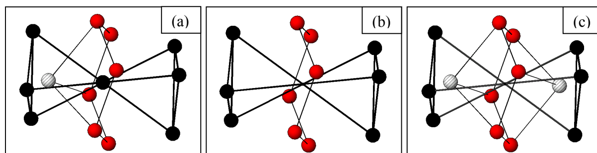
Figure I.17 : Environnement local du site 16d dans les pyrochlores \text{Pb}_{1+X}\text{Ta}_2\text{O}_{6+X} ( 1.33 \leq X \leq 1.6 ) [109] ; (a) cation \text{Pb}^{2+} en coordination pyramidale 1+6 ; (b) lacune [\text{Pb}^{2+}] en coordination 6 ; (c) lacune [\text{Pb}^{2+}] en coordination 2+6
