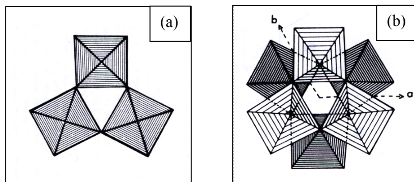
Figure I.2 : (a) unité structurale M_3O_{15} ; (b) unité structurale M_6O_{24}
