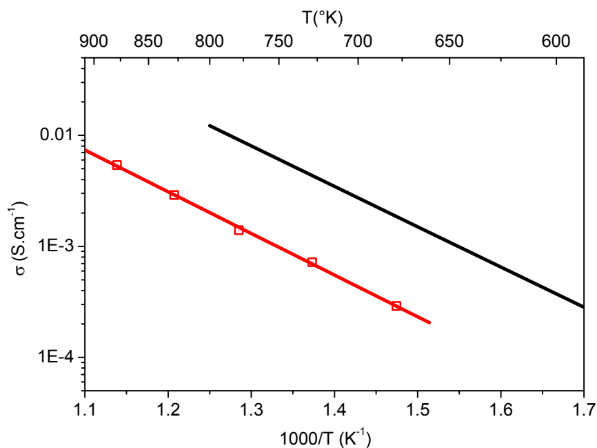
Figure IV.13 : Conductivité totale de Ce_{0.9}Gd_{0.1}O_{1.95} mesurée par impédance complexe à partir d'une pastille frittée (à droite) ou d'une pastille densifiée sous HP–MT (à gauche)
