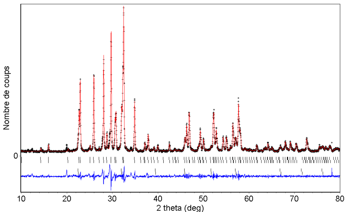
Figure IV.4 : Diffractogrammes X expérimental (croix) et calculé (ligne continue) de Sr_{1.5}Pb_{0.2}Ga_{0.3}Ta_{1.7}O_{6.4} recuit à 1000°C pendant 10h. Les positions des pics de Bragg dans la phase TTB et dans la phase perovskite ainsi que la fonction différence sont reportées de haut en bas.
