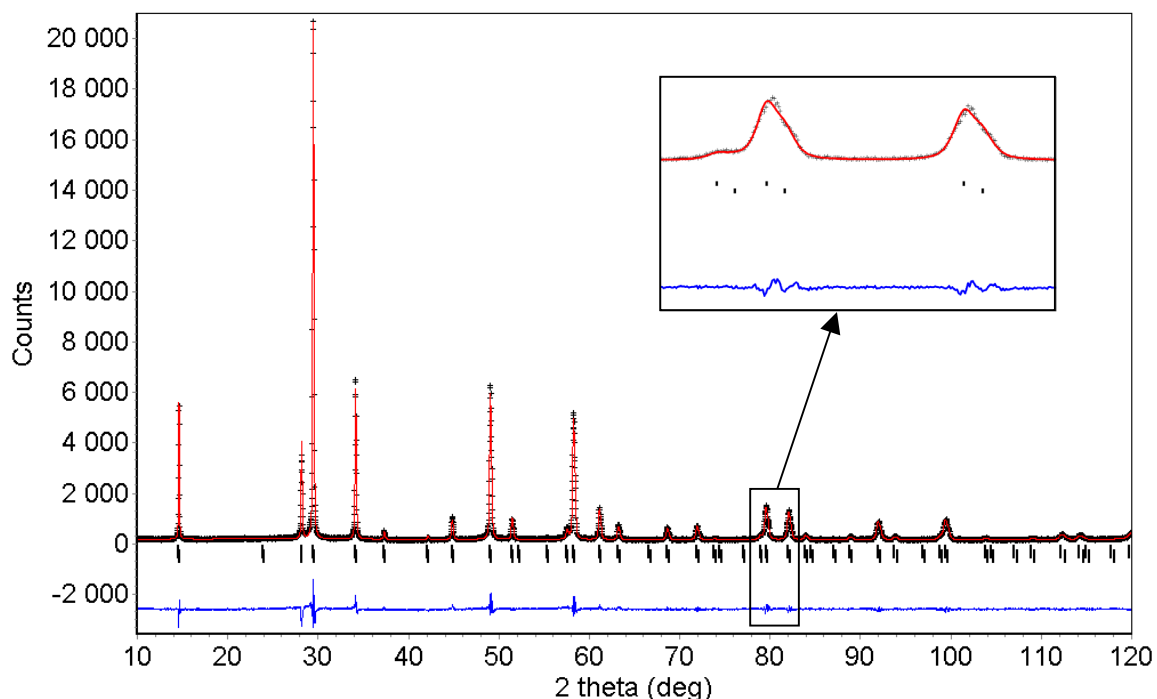
Figure III.4 : Diffractogramme X expérimental (croix) et calculé (ligne continue) de Sr_{1.5}Pb_{0.2}Ga_{0.3}Ta_{1.7}O_{6.4} , ainsi que leur fonction différence (en bas). Les positions des pics de Bragg sont également indiquées par des tirets verticaux
