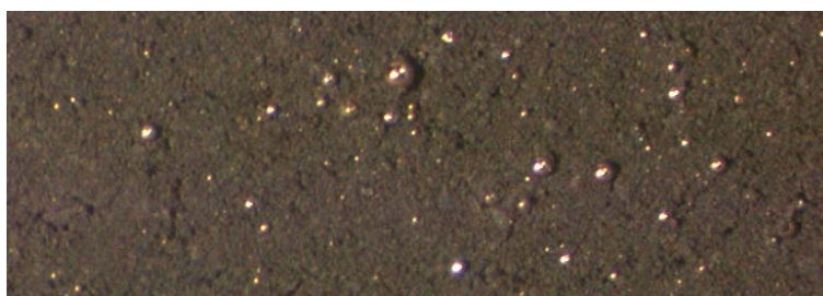
Figure II.1 : Grossissement (x10) des gouttelettes de plomb métallique dans la phase pyrochlore Pb_2Ga_{0.5}Ta_{1.5}O_{6.5} après traitements thermiques sous Ar/H_2 (5%)
