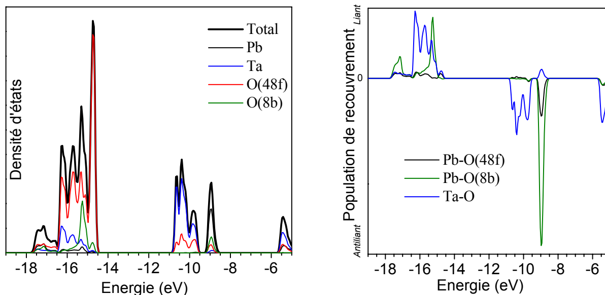
Figure II.8 : Courbes de densité d'états totales et partielles, et courbes de population de recouvrement pour " Pb_2Ta_2O_7 ", calculées par la méthode EHTB. La même échelle a été utilisée pour l'axe des populations de recouvrements dans les figures II.7 et II.8, afin de faciliter la comparaison des valeurs
