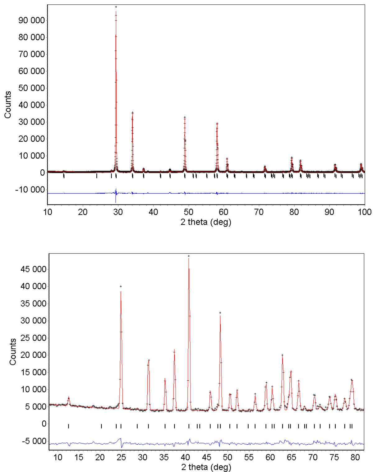
Figure III.1 : Diffractogrammes de rayons X (en haut) et de neutrons (en bas) expérimentaux (croix) et calculés (lignes continues) de Pb_2Ga_{0.5}Ta_{1.5}O_{6.5} , ainsi que leur fonction différence. Les positions des pics de Bragg sont également indiquées par des tirets verticaux
