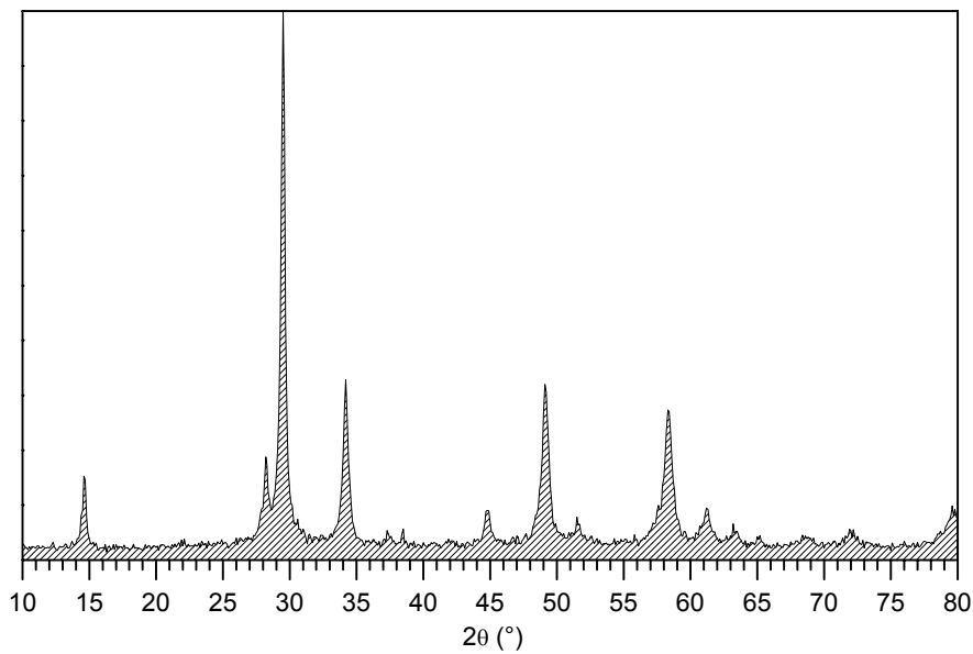
Figure IV.9 : Diffractogramme X d'une pastille de Pb_2Ga_{0.5}Ta_{1.5}O_{6.5} après réaction d'échange dans SrBr_2 et densification HP-MT
