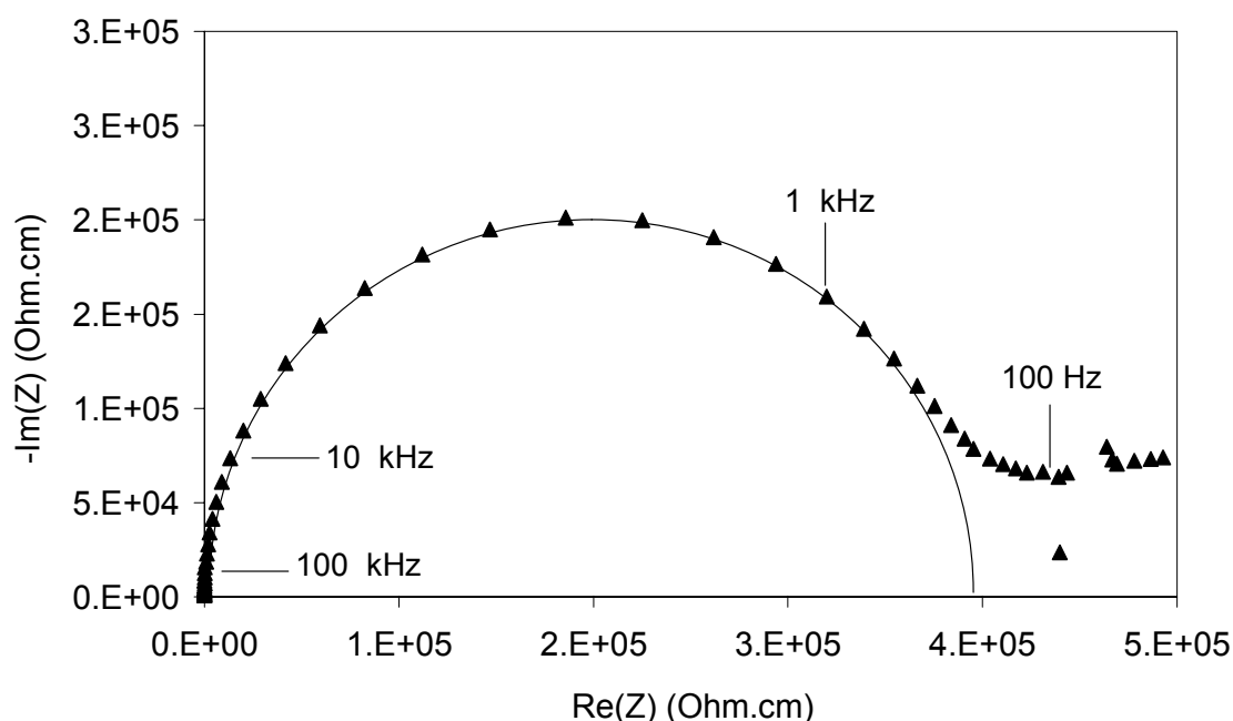
Figure IV.14 : Diagramme d’impédance, obtenu à 791°C, de Sr_{1.5}Pb_{0.2}Ga_{0.3}Ta_{1.7}O_{6.4} densifié sous HP–MT
