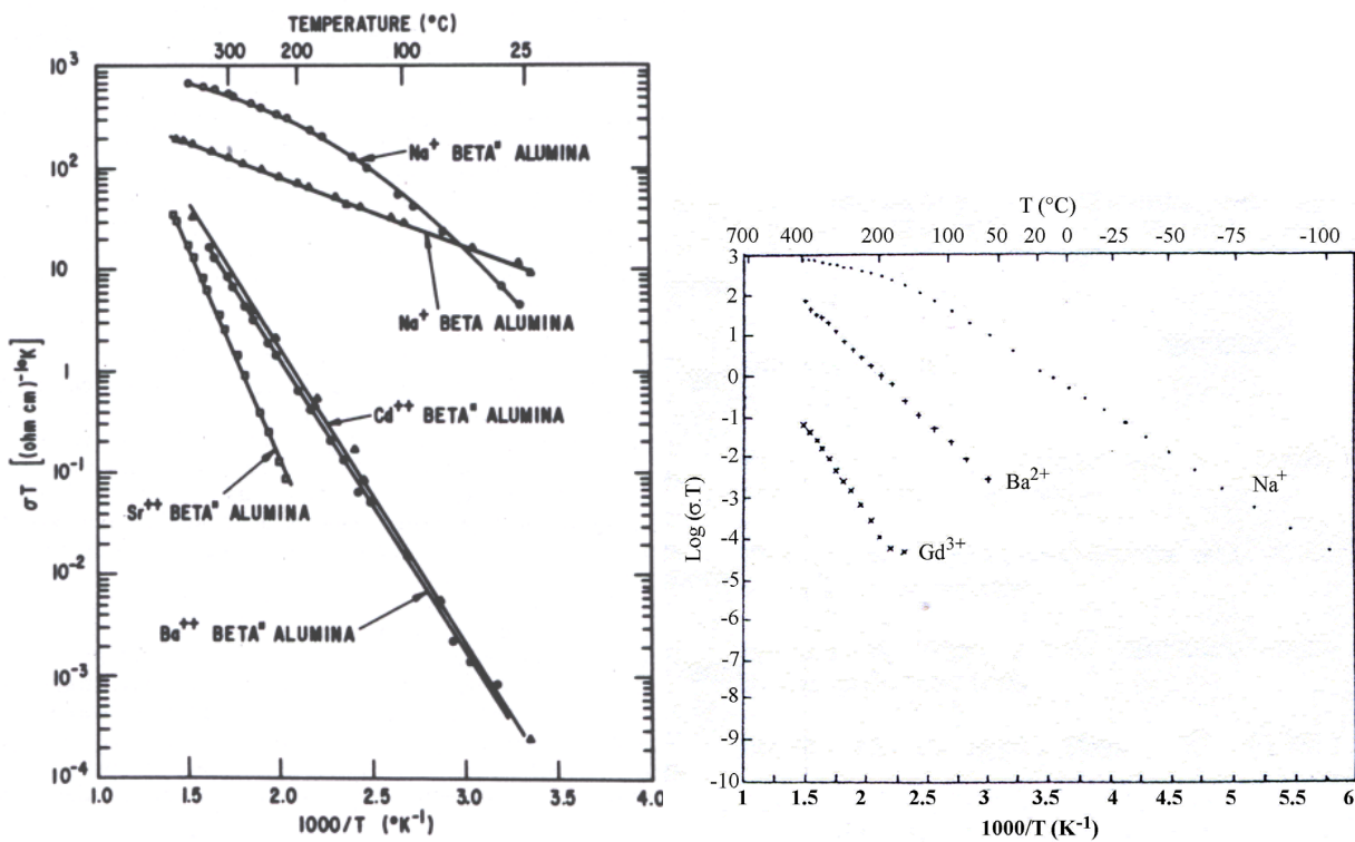
Figure I.10 : conductivité des ions Na^+ , Sr^{2+} , Ba^{2+} , Cd^{2+} et Gd^{3+} dans les alumines \beta et \beta'' [60,61]
