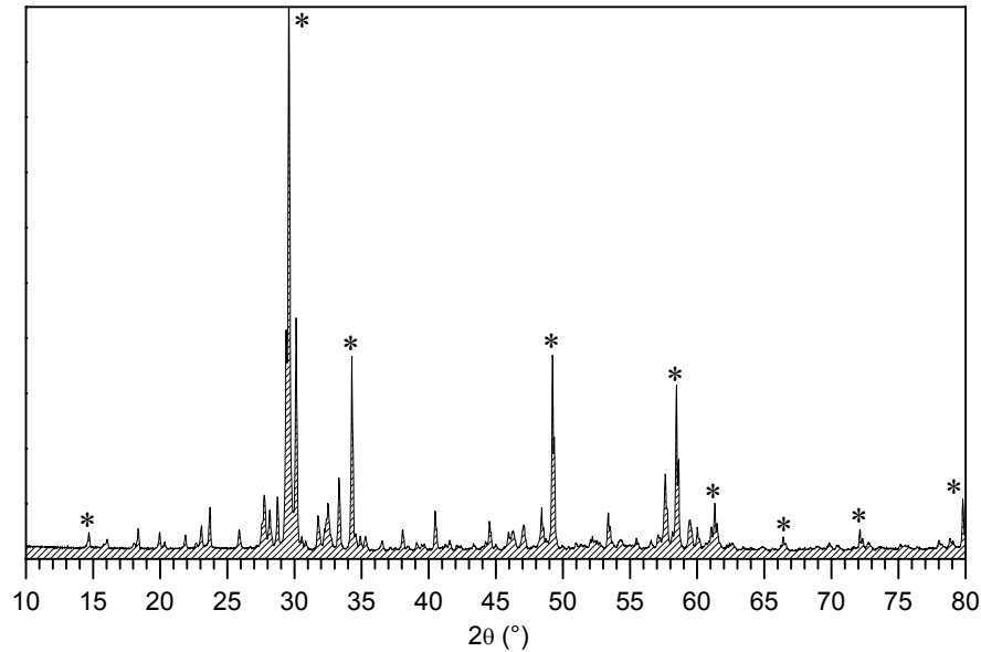
Figure IV.6 : Diffractogramme X de Nd_{1.1}Pb_{0.35}Ga_{0.5}Ta_{1.5}O_{6.5} recuit sous air à 1100^{\circ}C (*, phase de structure pyrochlore)
