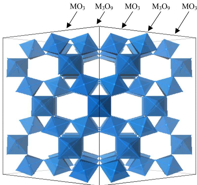
Figure I.16 : Vue suivant l'axe [110] du mode d'empilement de type ABC des couches M_3O_9 et MO_3 au sein du réseau pyrochlore.
