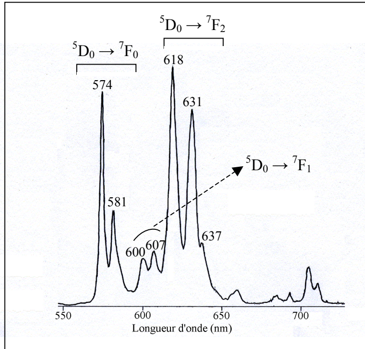
Figure III.14 : Spectre d'émission (intensité en unités arbitraires) de La_{1.1}Pb_{0.35}Ga_{0.5}Ta_{1.5}O_{6.5}(Eu) entre 550 et 750 nm sous excitation par \lambda = 254 nm
