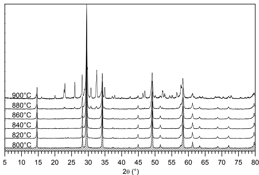
Figure IV.3 : Diffractogrammes X de Sr_{1.5}Pb_{0.2}Ga_{0.3}Ta_{1.7}O_{6.4} recuit sous air à températures croissantes.
