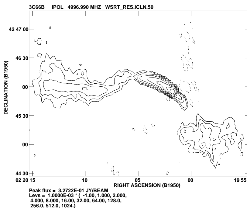
Figure 1: Carte de 3C66B à 5 secondes d'arc de résolution avec l'interféromètre de Westerbork.
