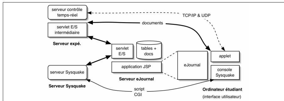
Figure 3. Architecture multi-serveurs d'un cockpit pour un cours d'automatique
